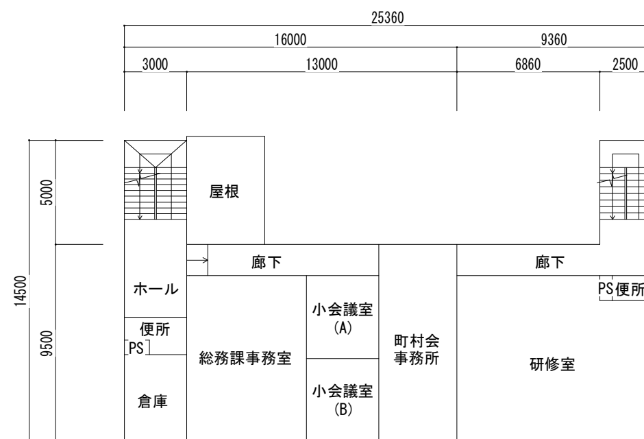
2階平面図
