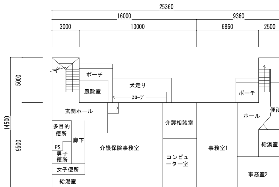
1階平面図
