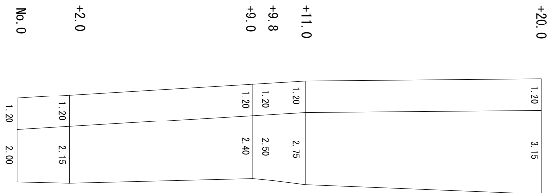
舗装展開図 S=1:100
