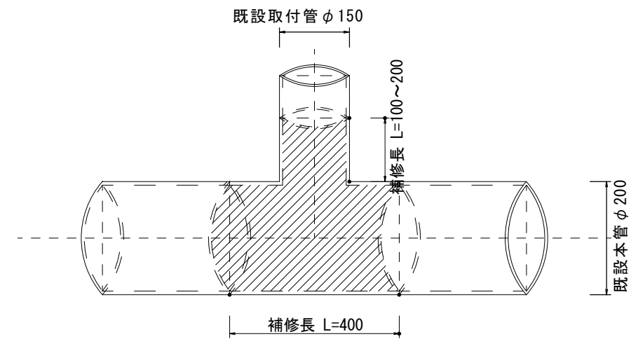
支管一体部分補修工
