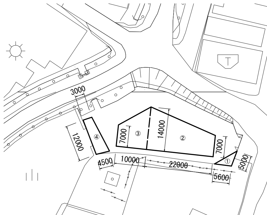
平面図 S=1/500
