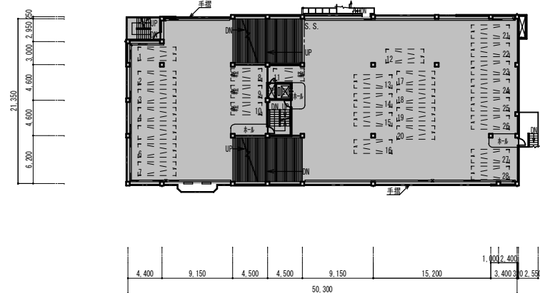
3階平面図
