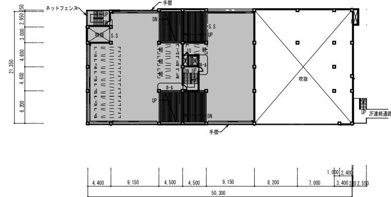
2階平面図
