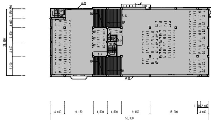
4階平面図
