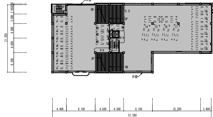
7階平面図
