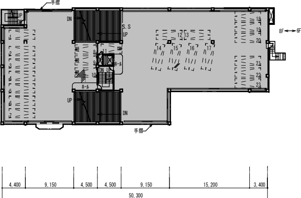
8階平面図
