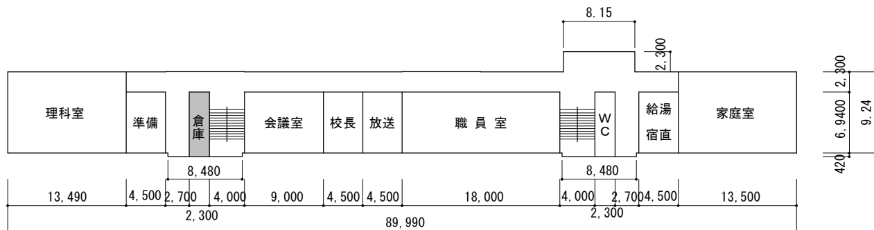
1階平面図
