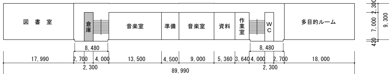
3階平面図
