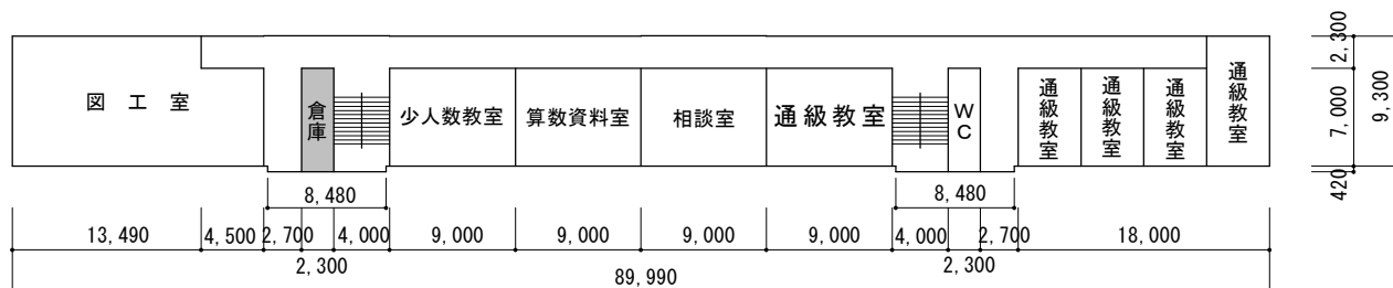
2階平面図
