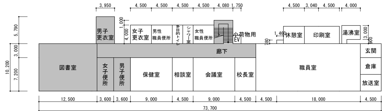
1 階平面図
