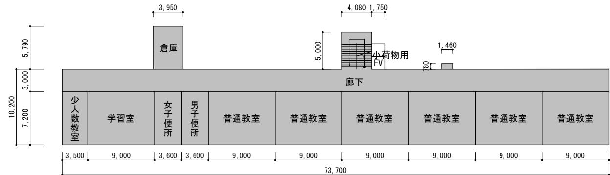
2 階平面図
