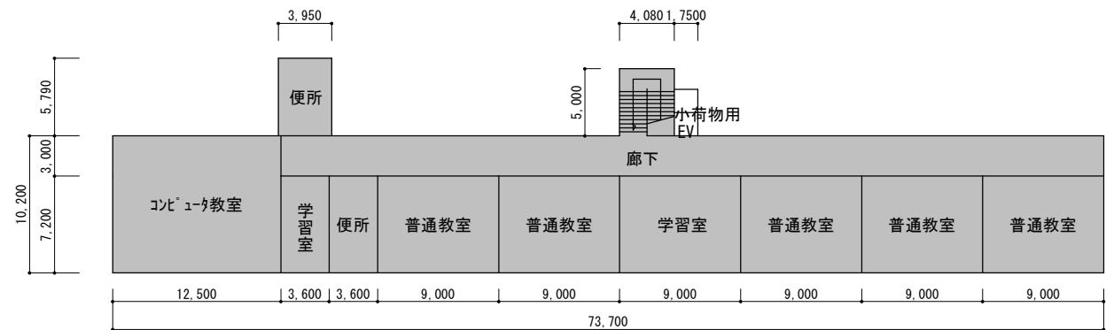
3 階平面図
