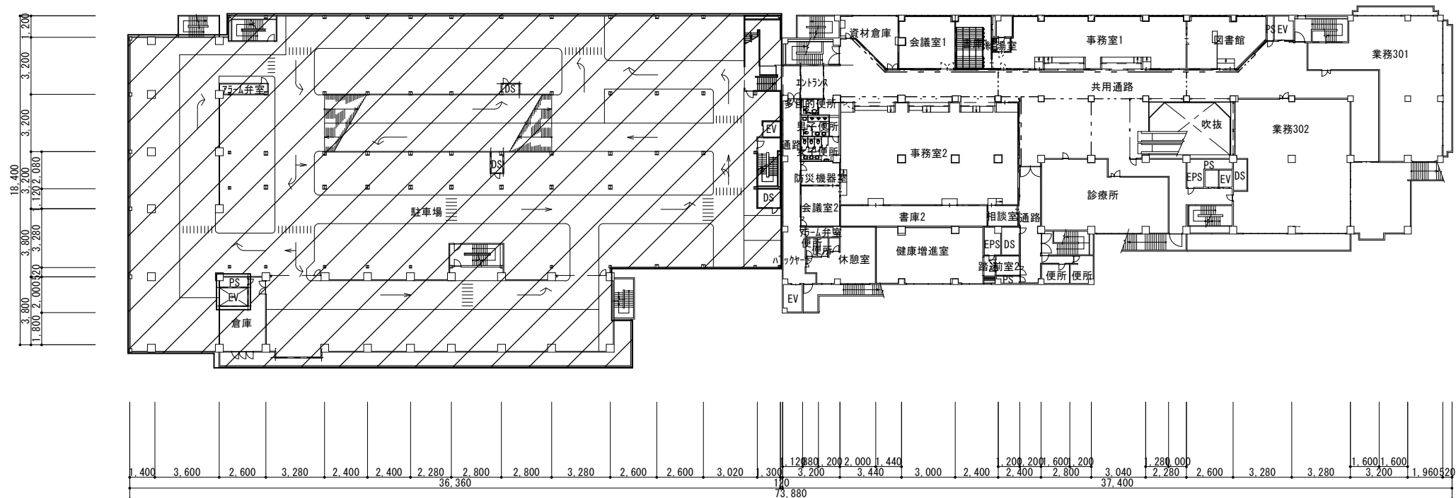
3 階平面図
