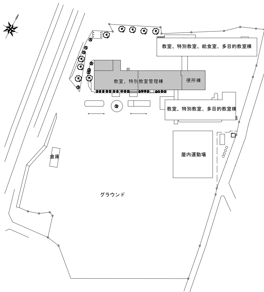
配置図
