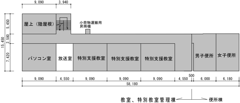
2 階平面図
