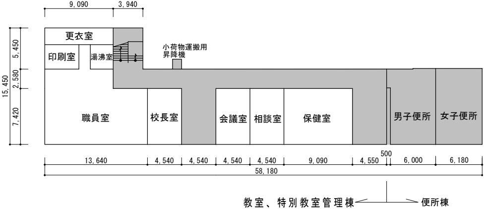
1 階平面図
