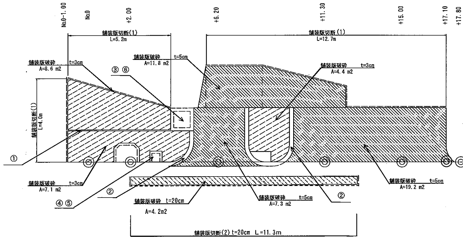
舗装取壊し平面図
