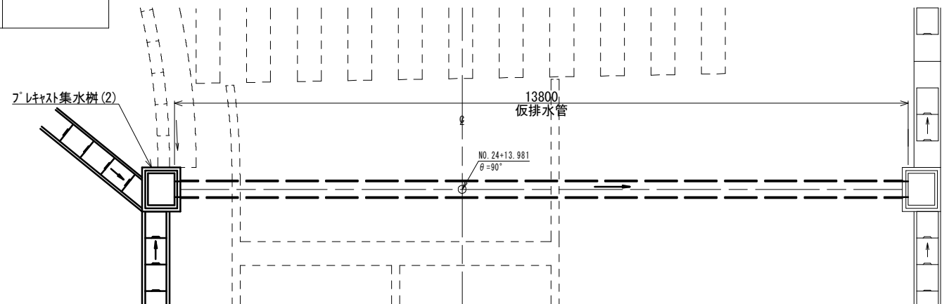
平面図
