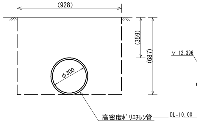
仮排水管 10.0m当り
