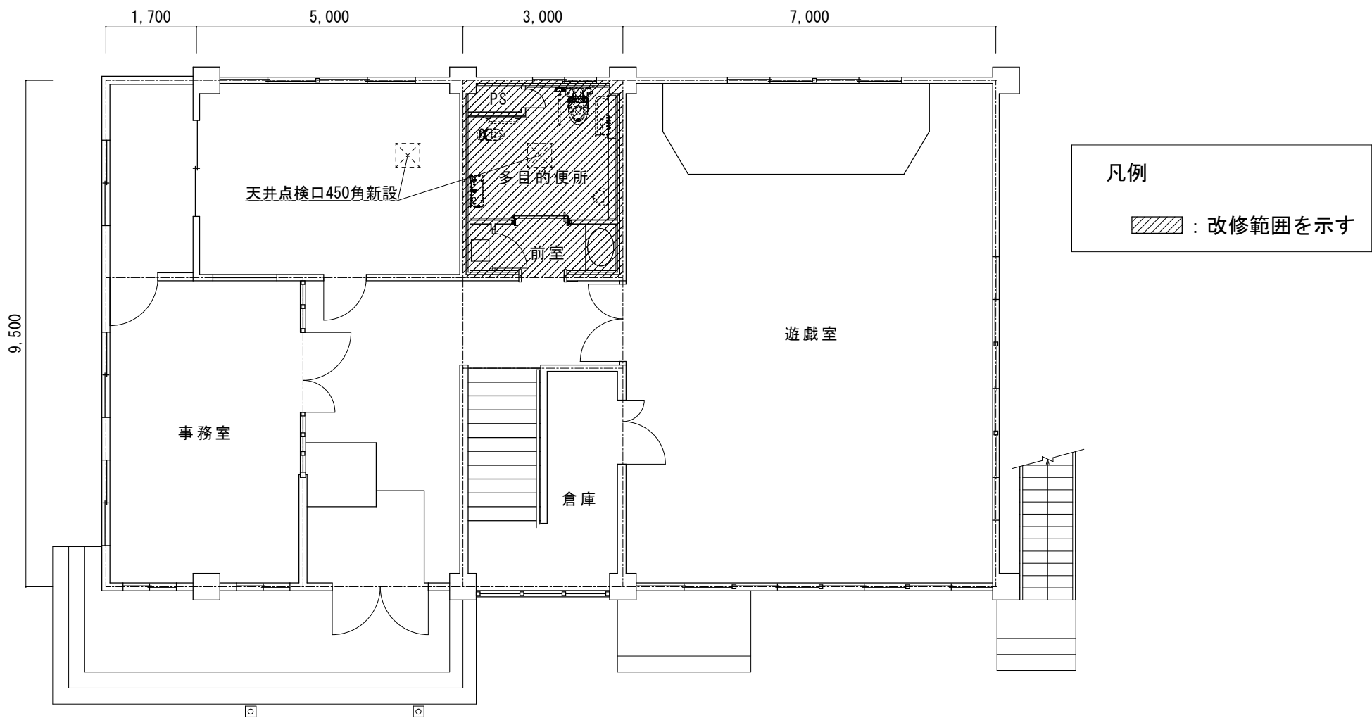
改修後 1 階平面図 S=1/100
