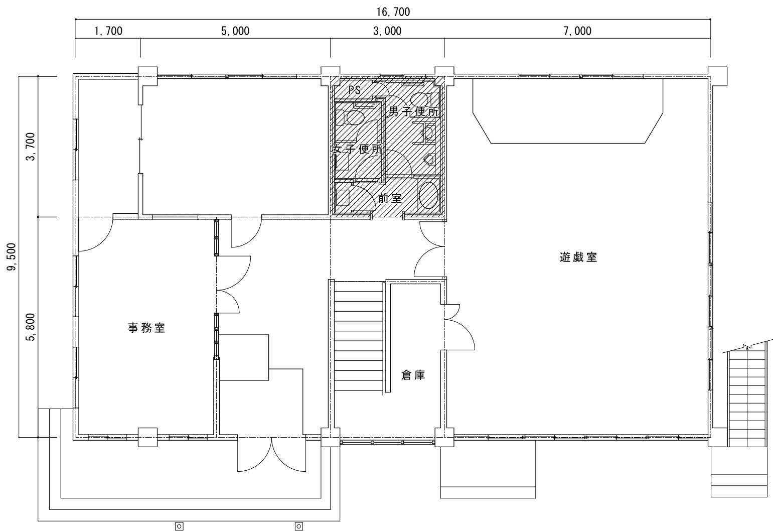
改修前 1 階平面図 S=1/100
