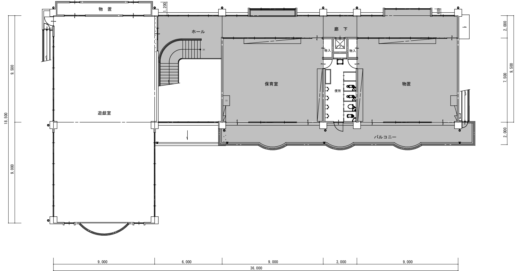
2階平面図
