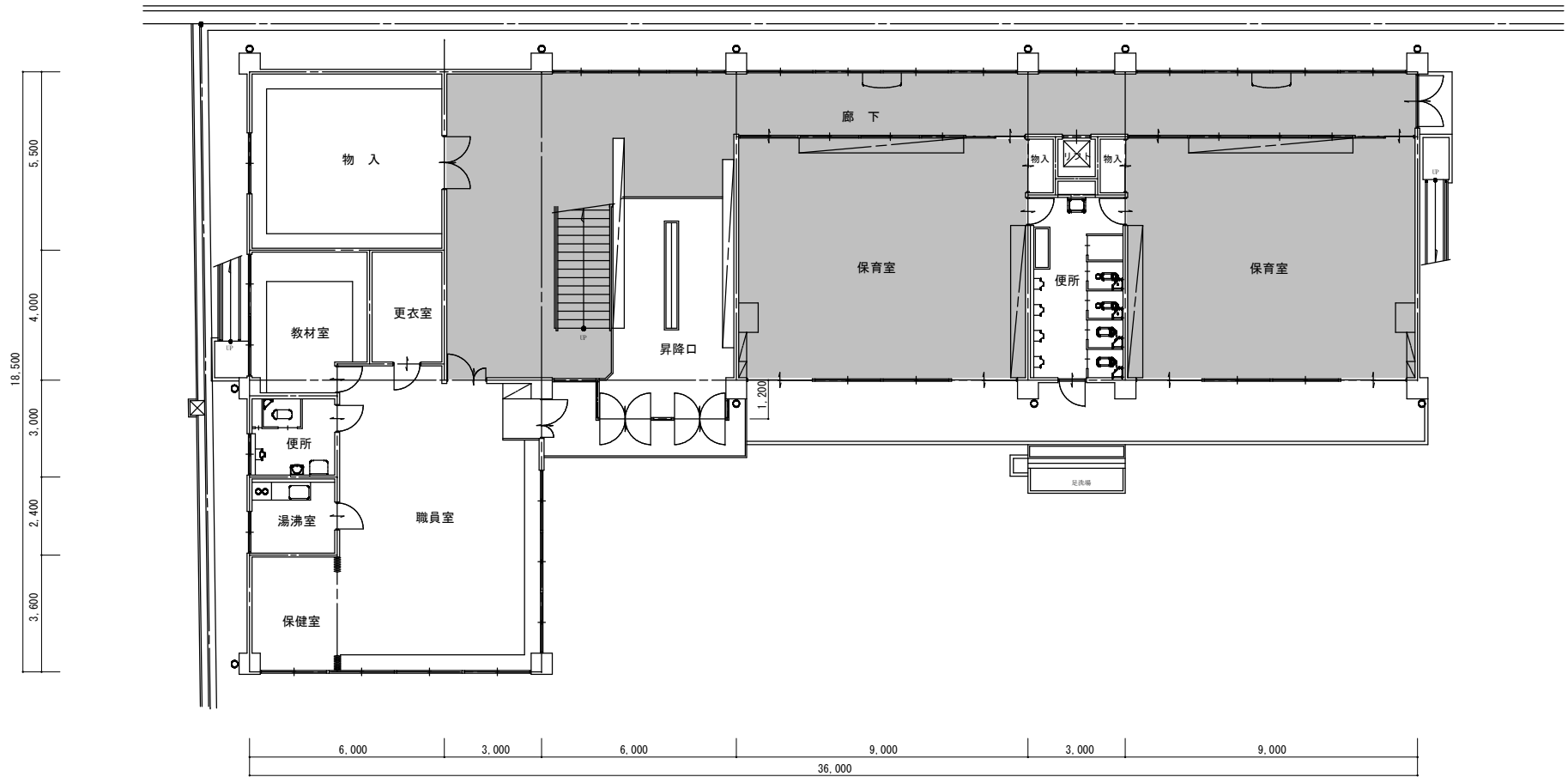
1階平面図
