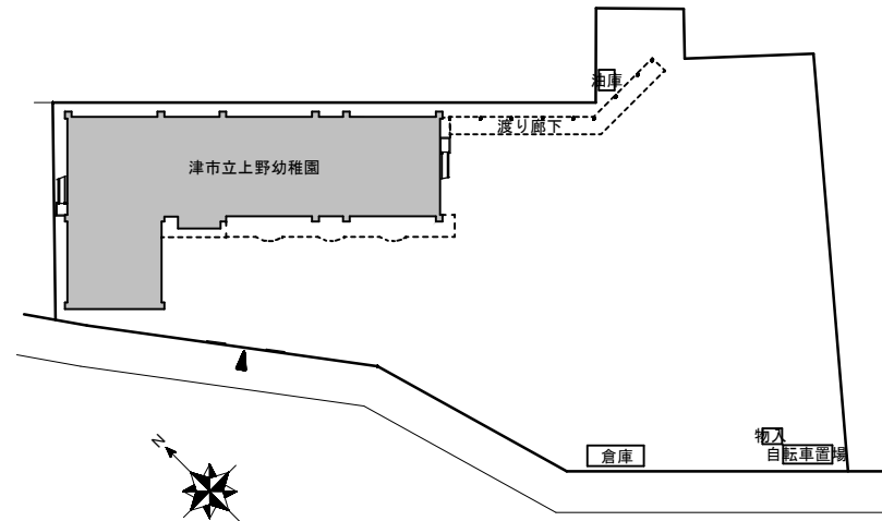
配置図
