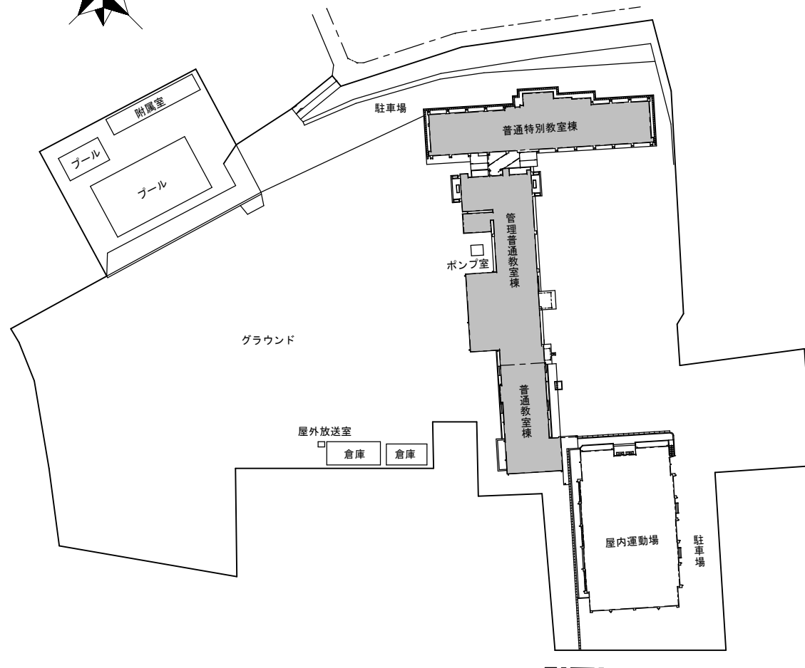
配置図
