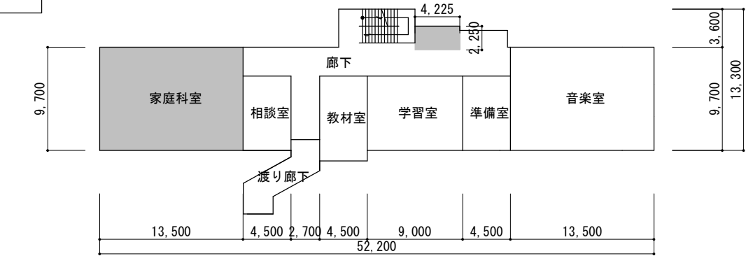
3 階 平面図
