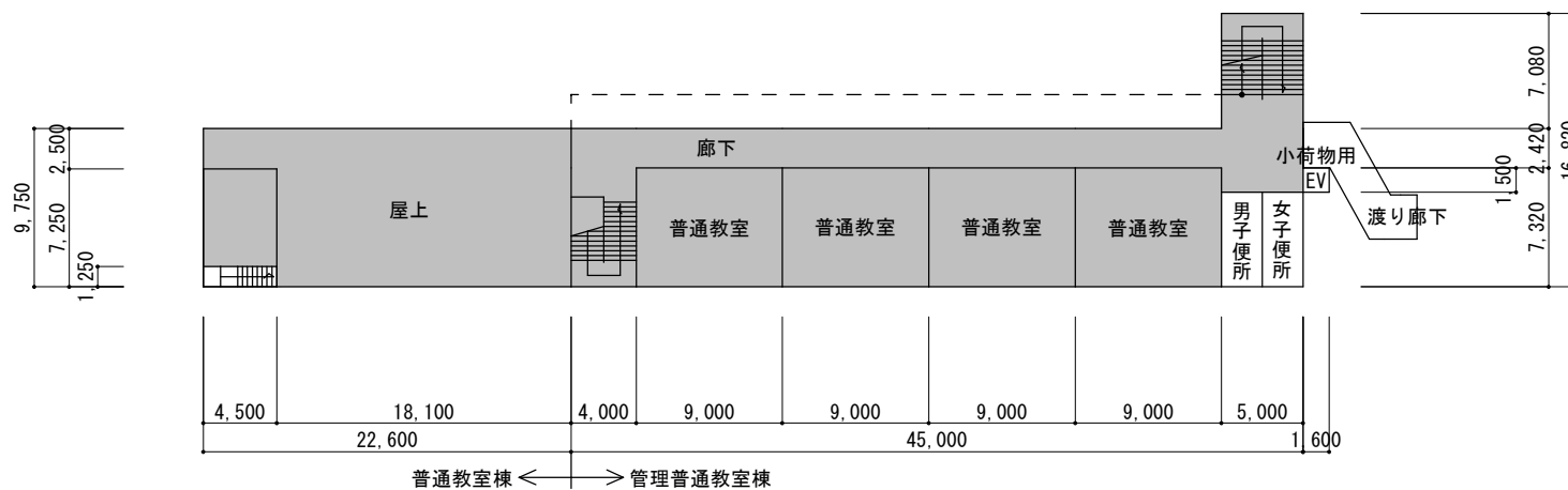
3 階平面図
