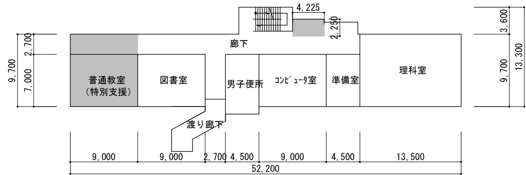
2 階 平面図
