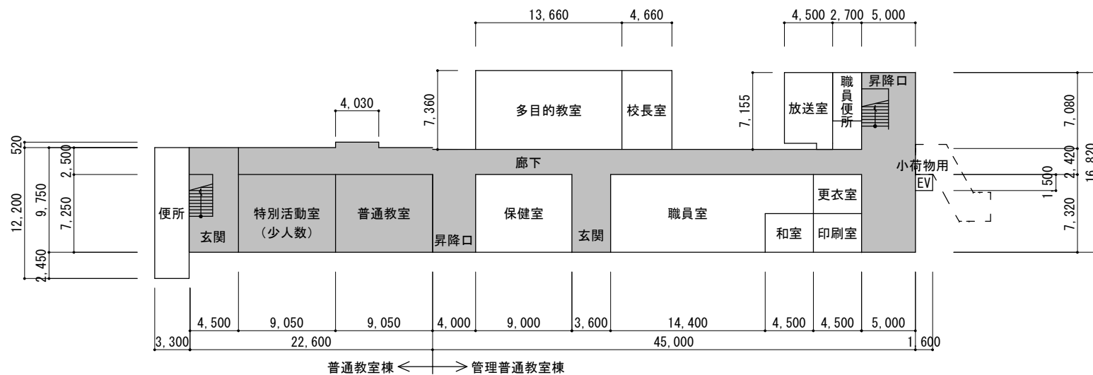
1 階平面図
