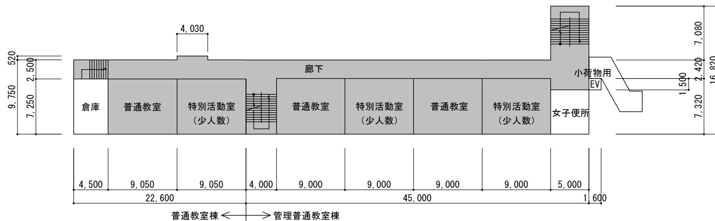
2 階平面図
