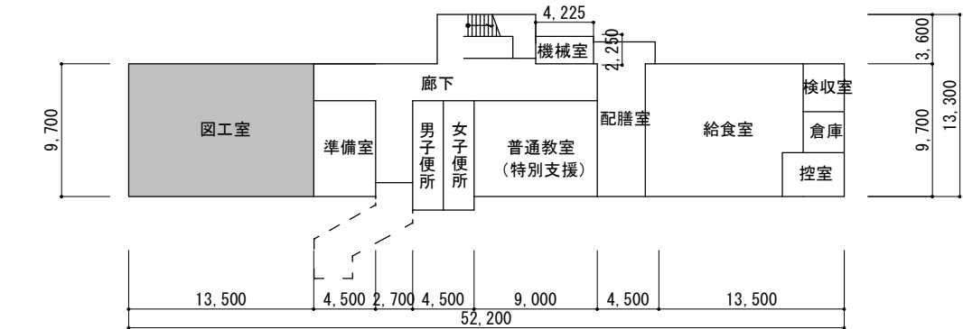
1 階 平面図
