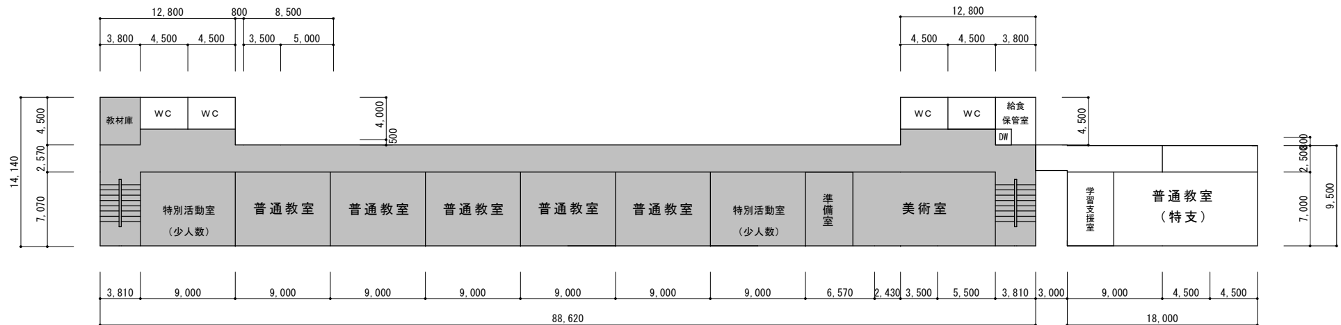
3 階平面図
