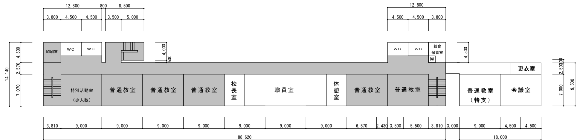
2 階平面図
