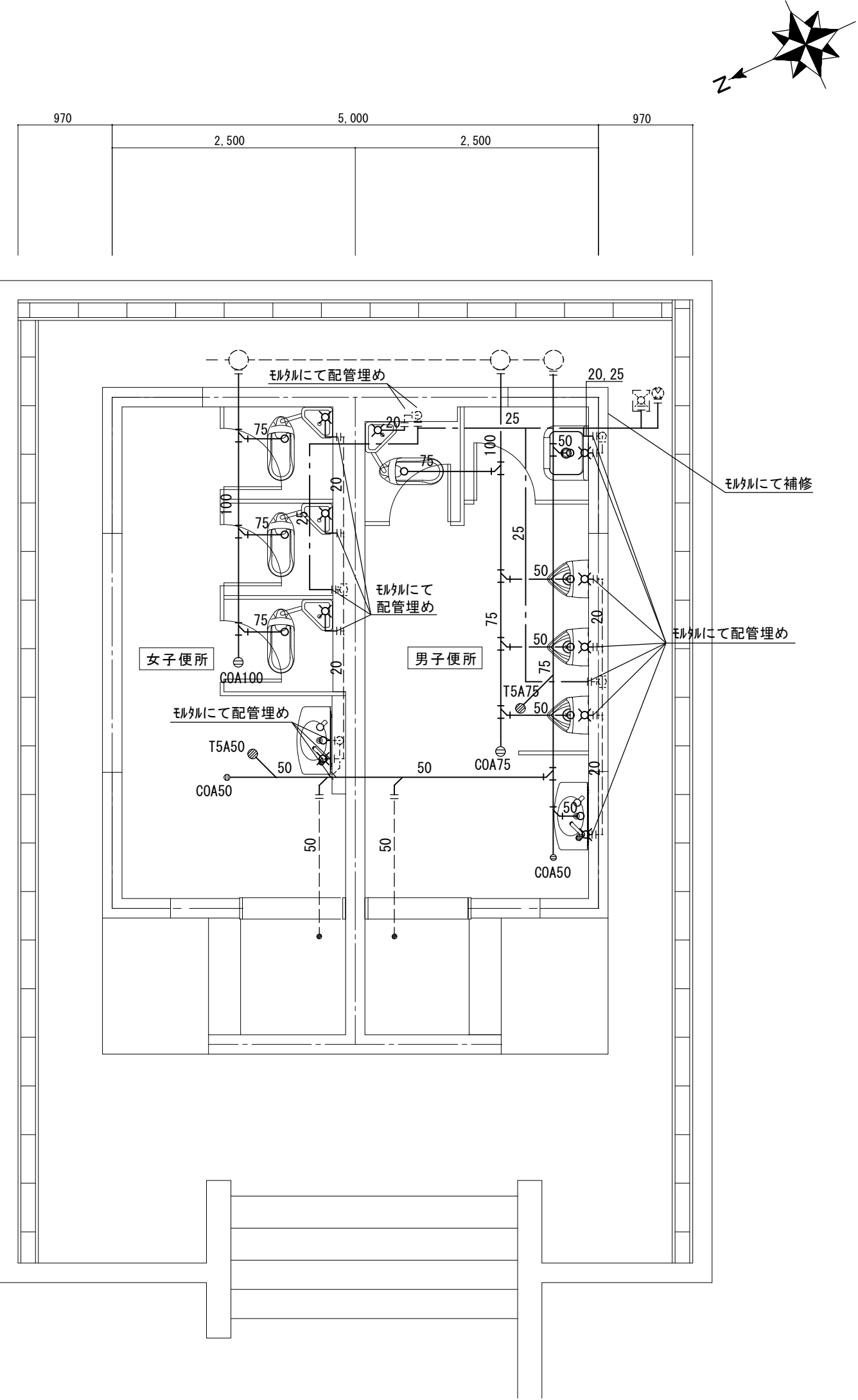
改修前 平面詳細図 S=1/50
