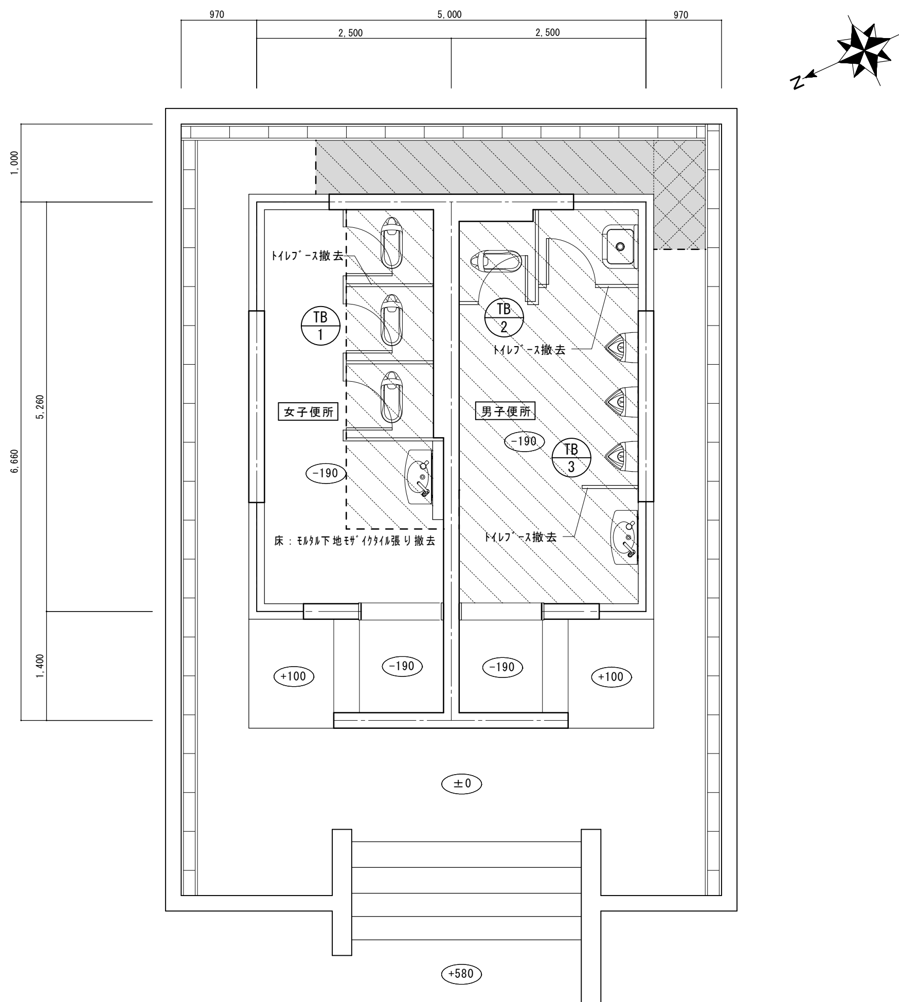
改修前 平面詳細図 S=1/50
