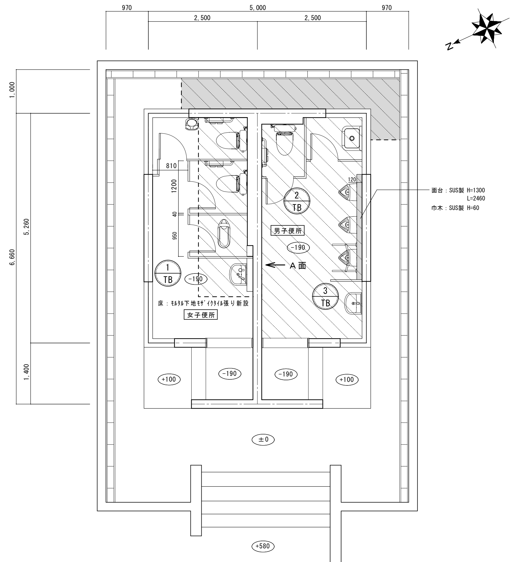
改修後 平面詳細図 S=1/50
