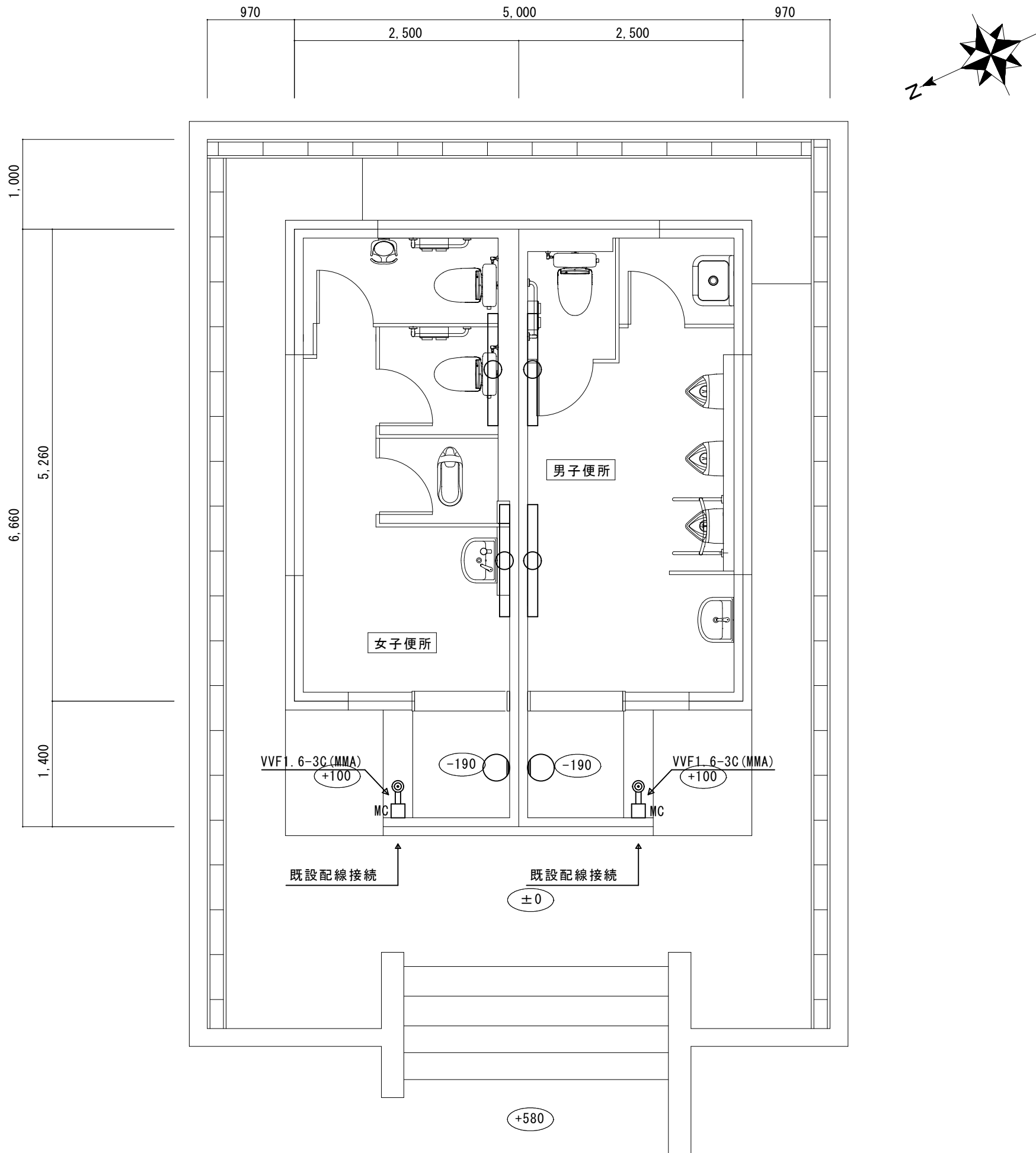
改修後 平面詳細図 S=1/50
