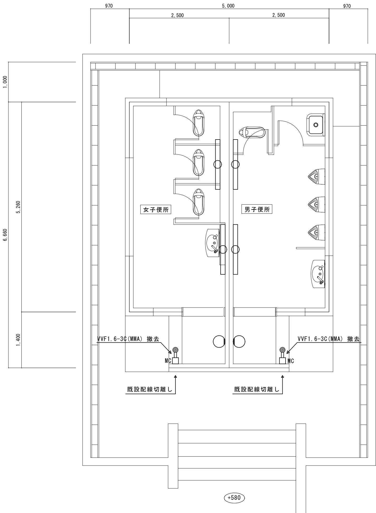
改修前 平面詳細図 S=1/50
