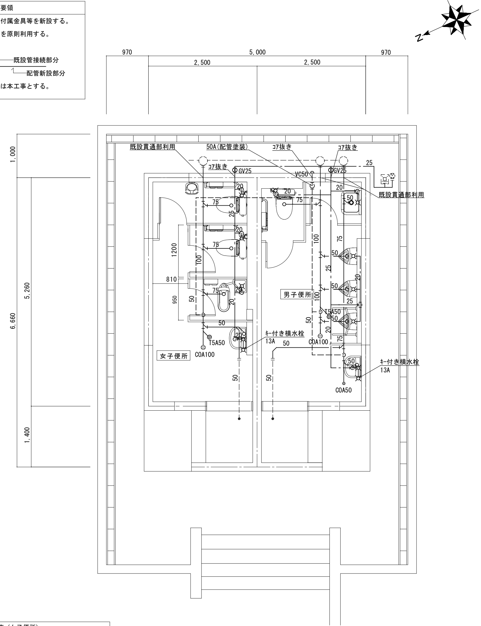
改修後 平面詳細図 S=1/50
