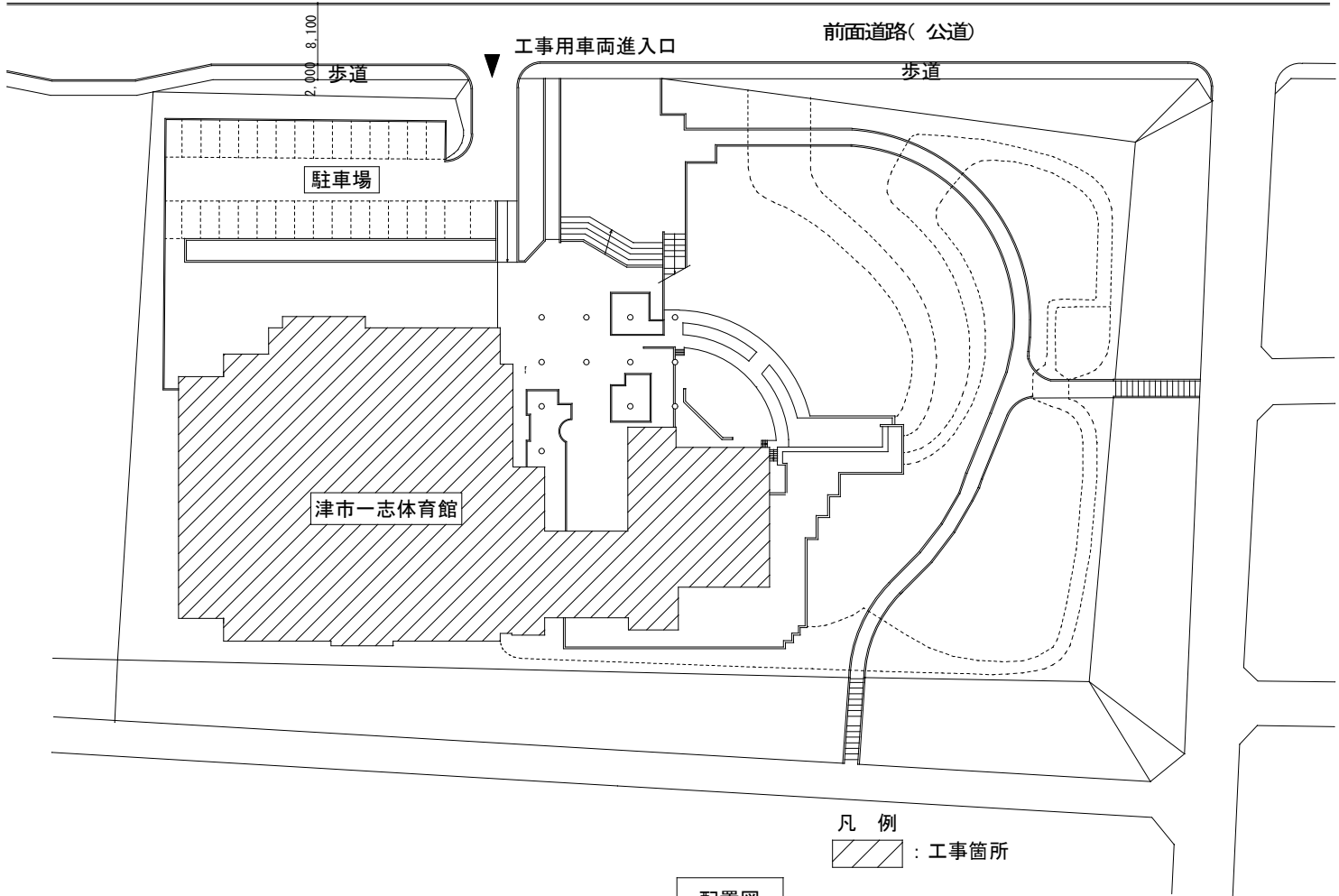
配置図
