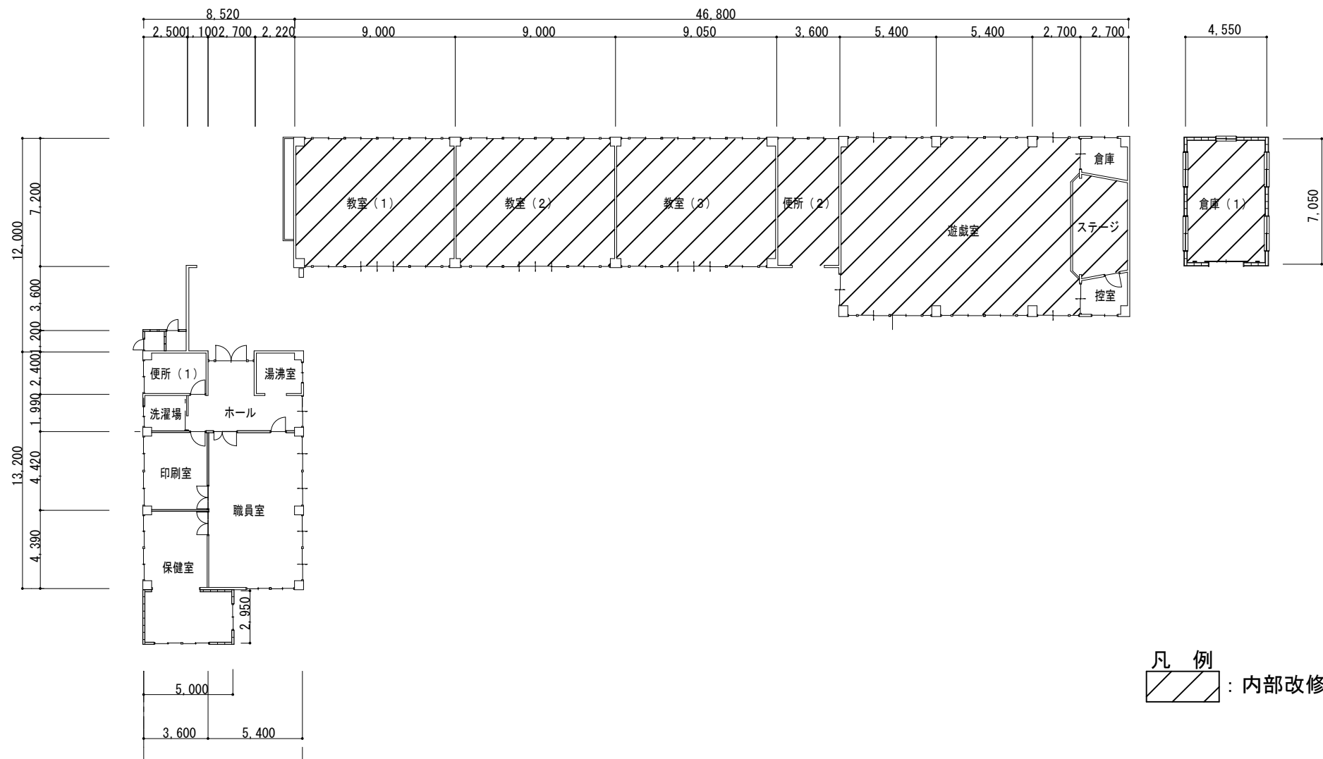
1 階平面図
