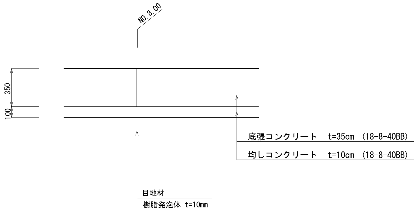
底張コンクリート詳細図
