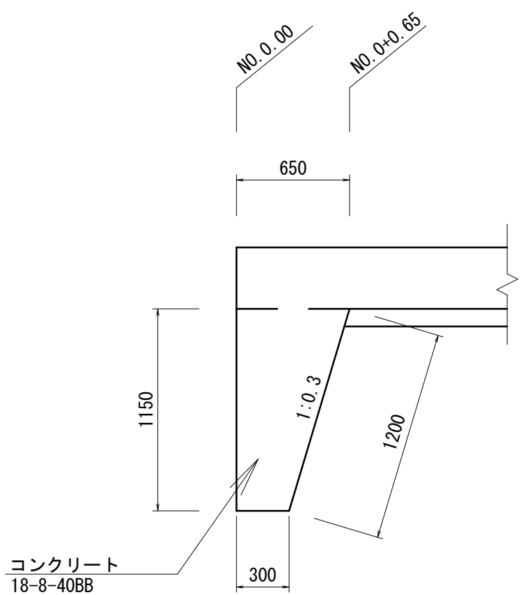
カットオフ部
