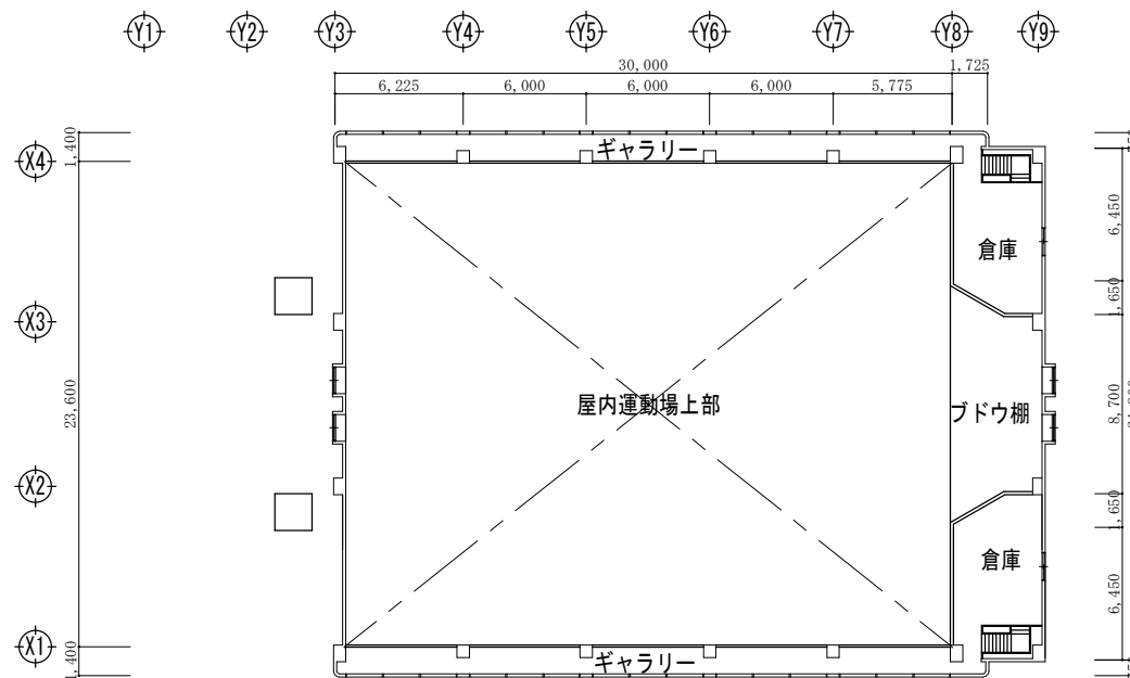
2 階平面図
