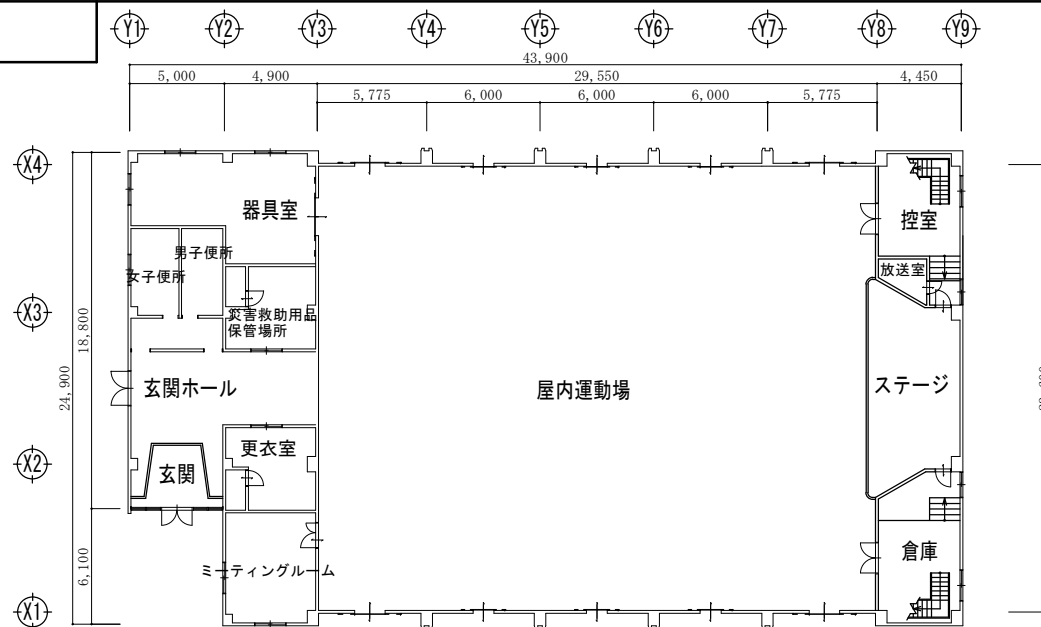
1 階平面図
