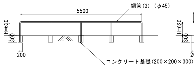
詳細断面図
