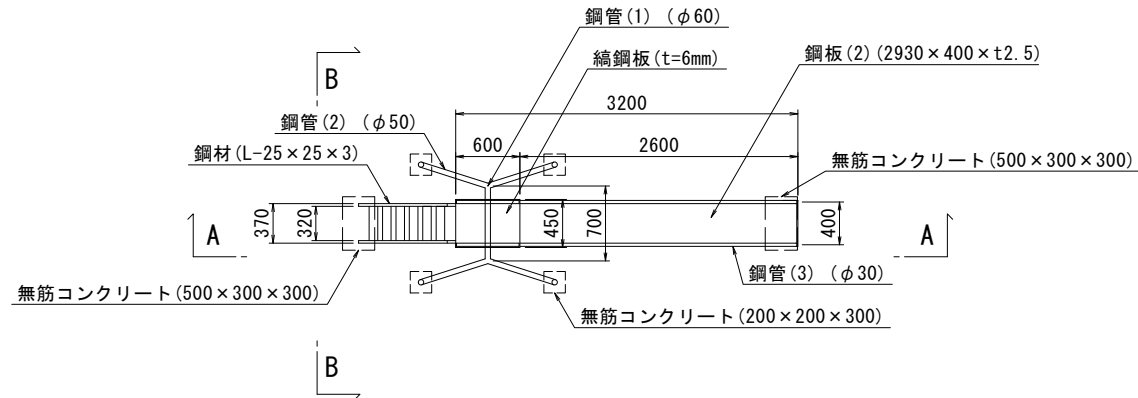
平面図
