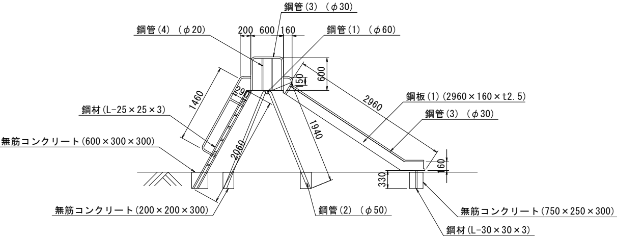
A - A
