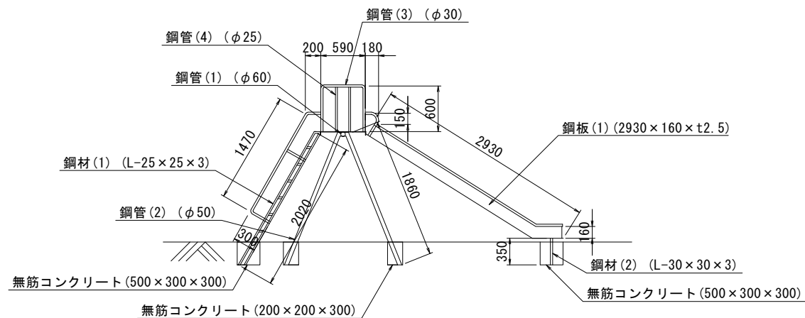
A - A
