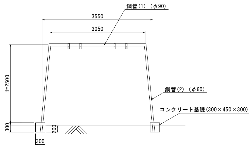
ブランコ正面図
