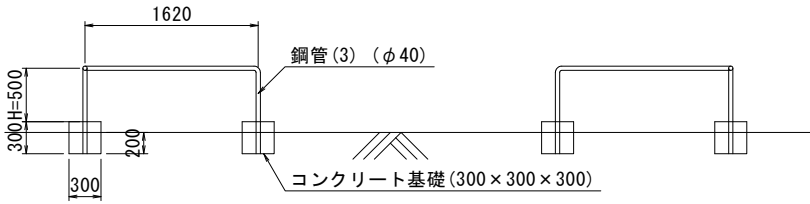
柵断面図
