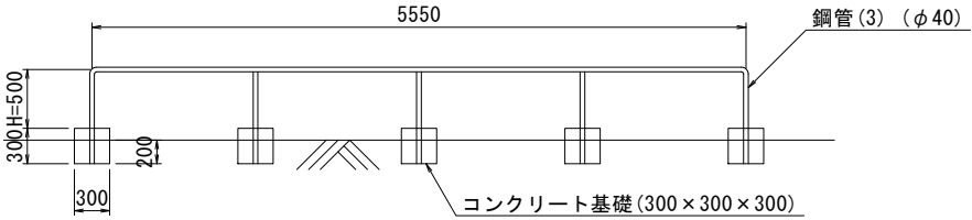
柵断面図
