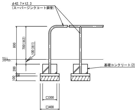
詳細図 S=1:20
