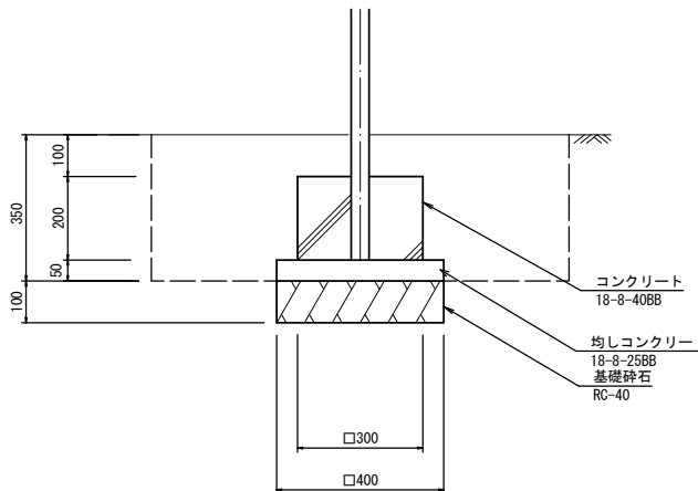
基礎コンクリート(4) S=1:10
