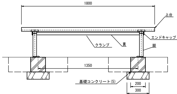
立面図 S=1:15
