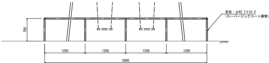
立面図 S=1:30
