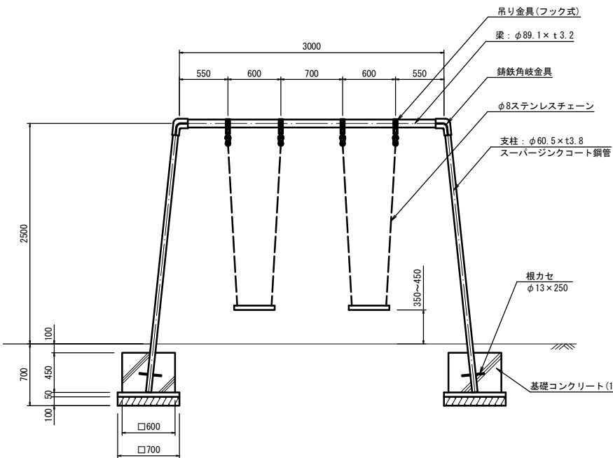
立面図 S=1:30
