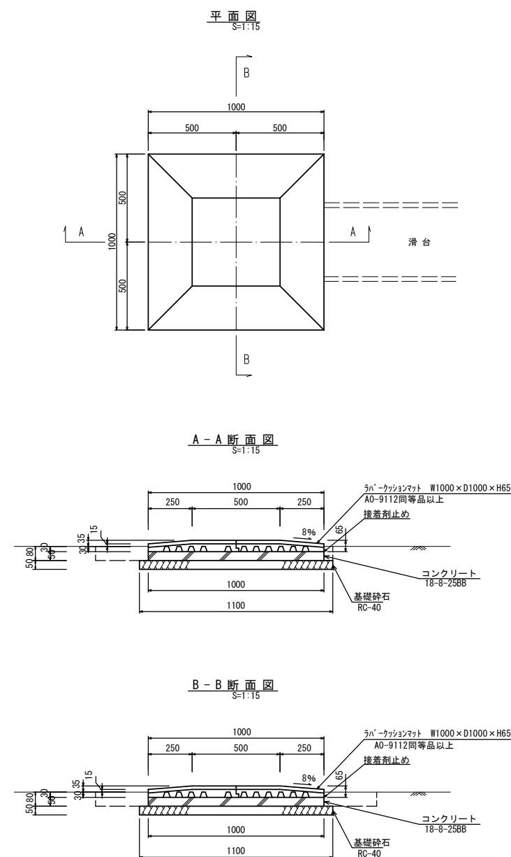
安全マット(2)詳細図 滑台用(A0-9112同等品以上)
