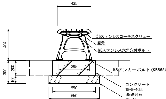
側面図 S=1:15
