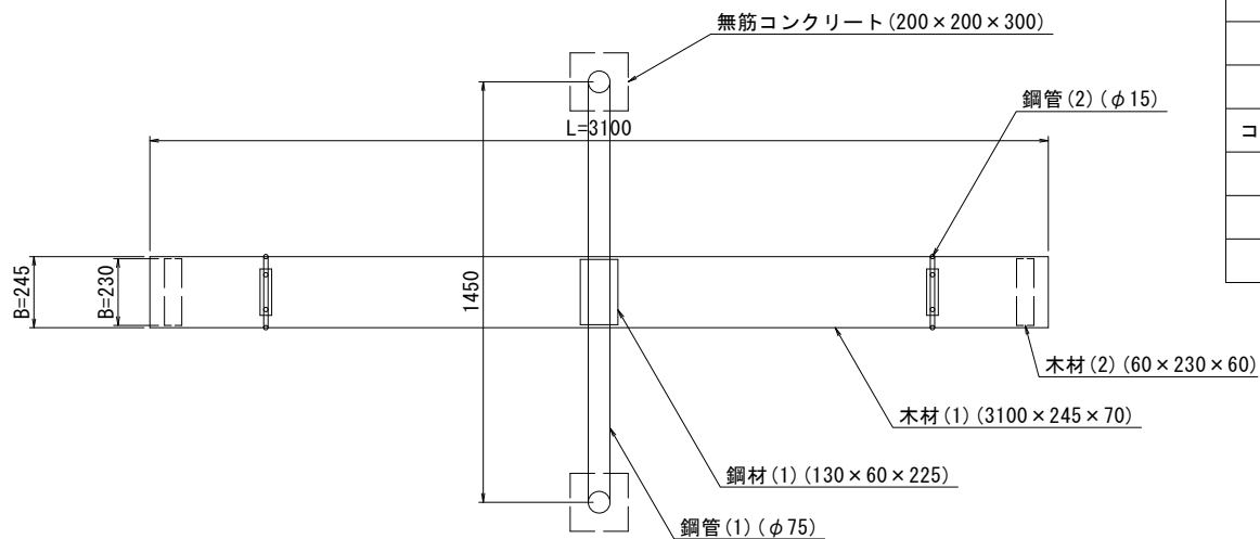
平面図
