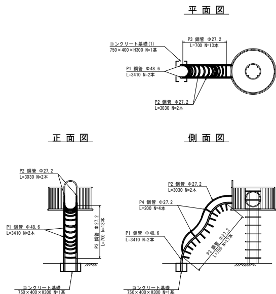
複合遊具撤去詳細図① S=1:50
