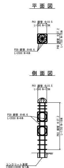
複合遊具撤去詳細図⑫ S=1/50
