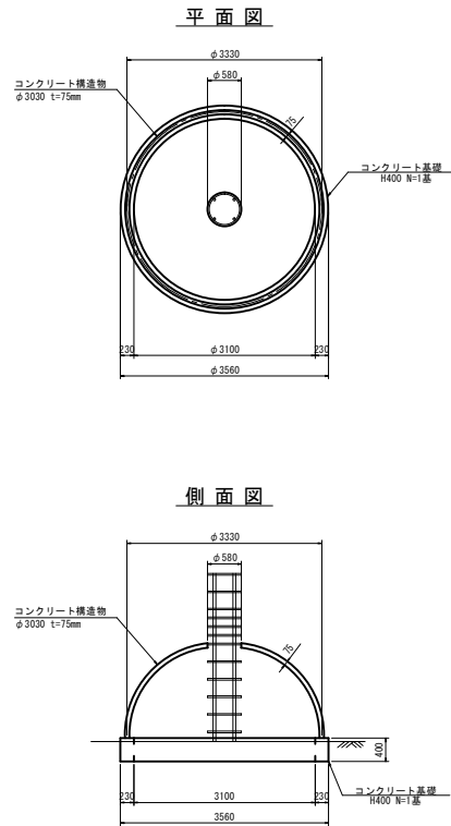
複合遊具撤去詳細図⑤ S=1/50
