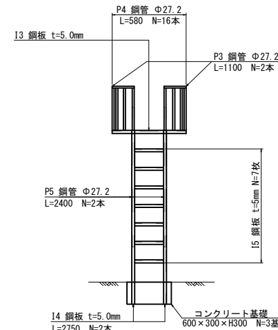
背面図
