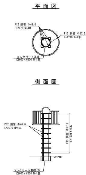
複合遊具撤去詳細図③ S=1:50
