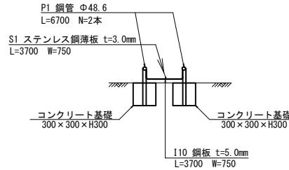
背面図
