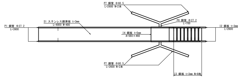
平面図 S=1:25
