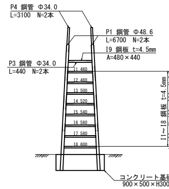
背面図
