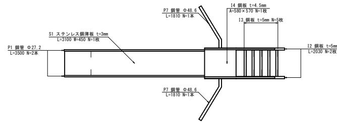
側面図 S=1:25
