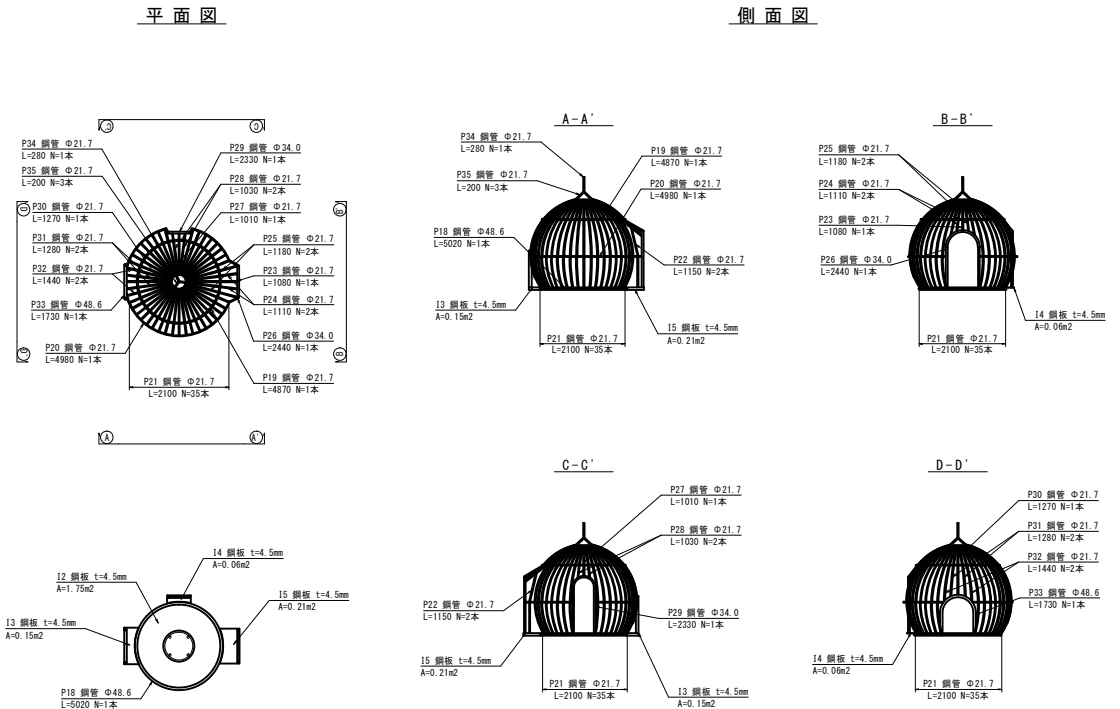
複合遊具撤去詳細図⑦ S=1/50
