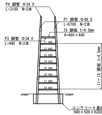
背面図
