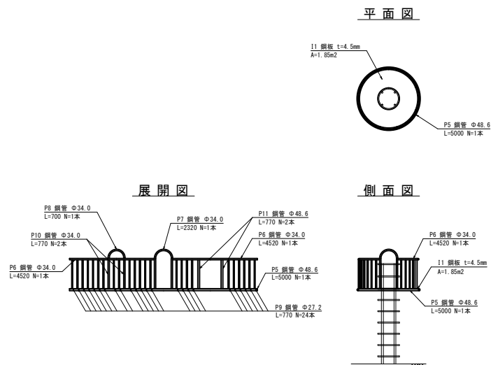
複合遊具撤去詳細図② S=1:50
