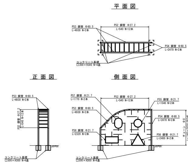
複合遊具撤去詳細図⑪ S=1/50
