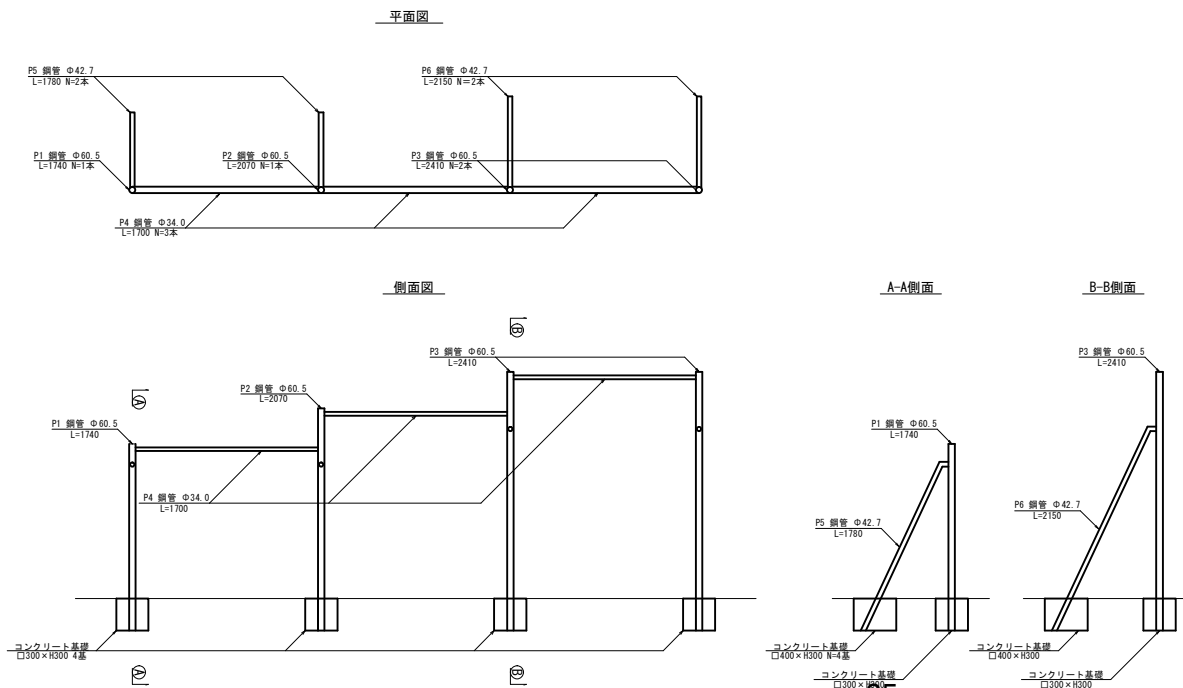
鉄棒(2)撤去構造図
