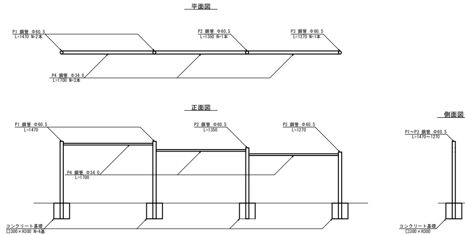
鉄棒(2)撤去構造図
