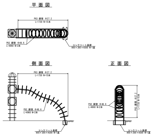
複合遊具撤去詳細図⑬ S=1/50
