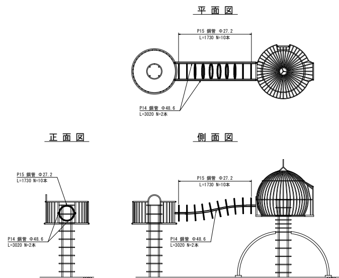
複合遊具撤去詳細図④ S=1:50
