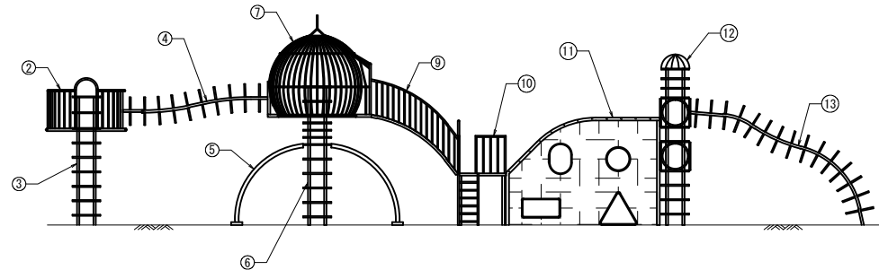
側面図 S=1/50
