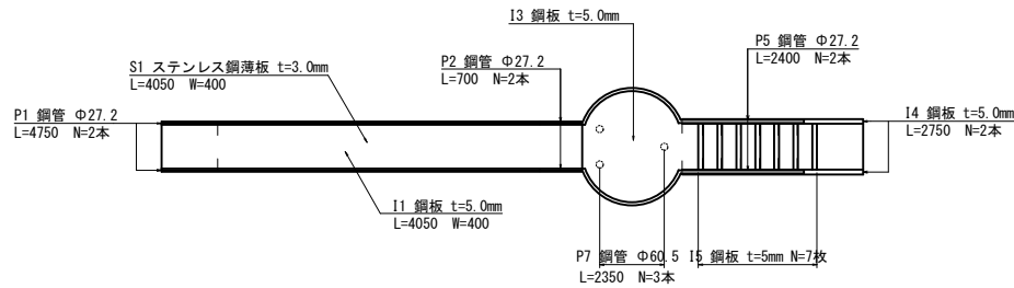
側面図
