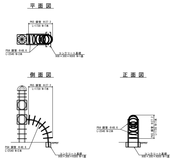
複合遊具撤去詳細図⑭ S=1/50
