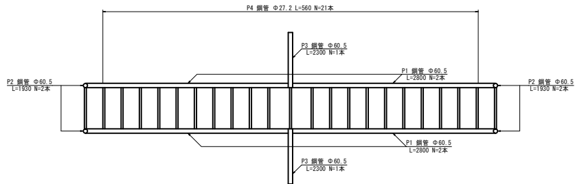
側面図
