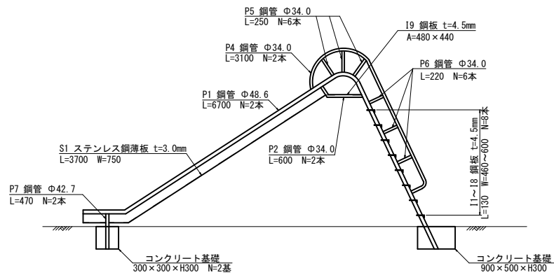
側面図
