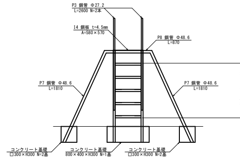
背面図 S=1:25
