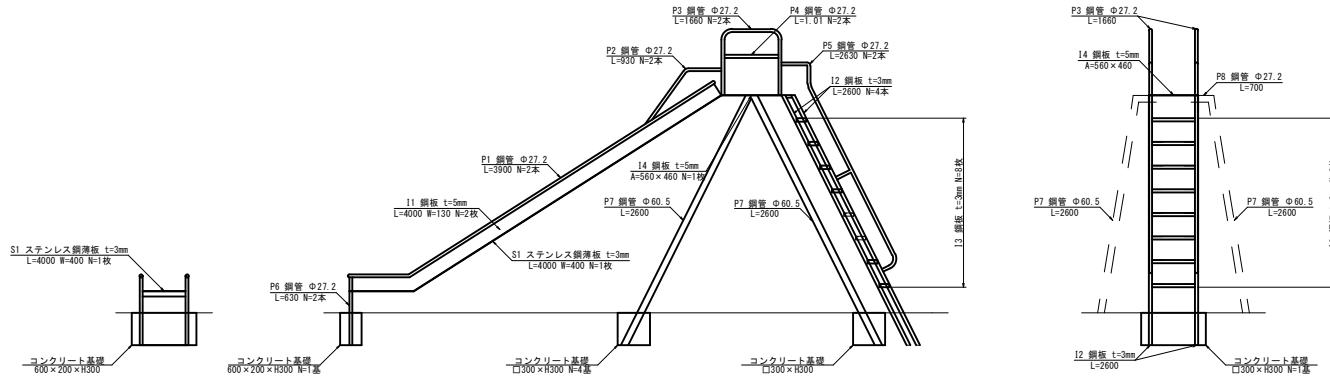
正面図 S=1:25
