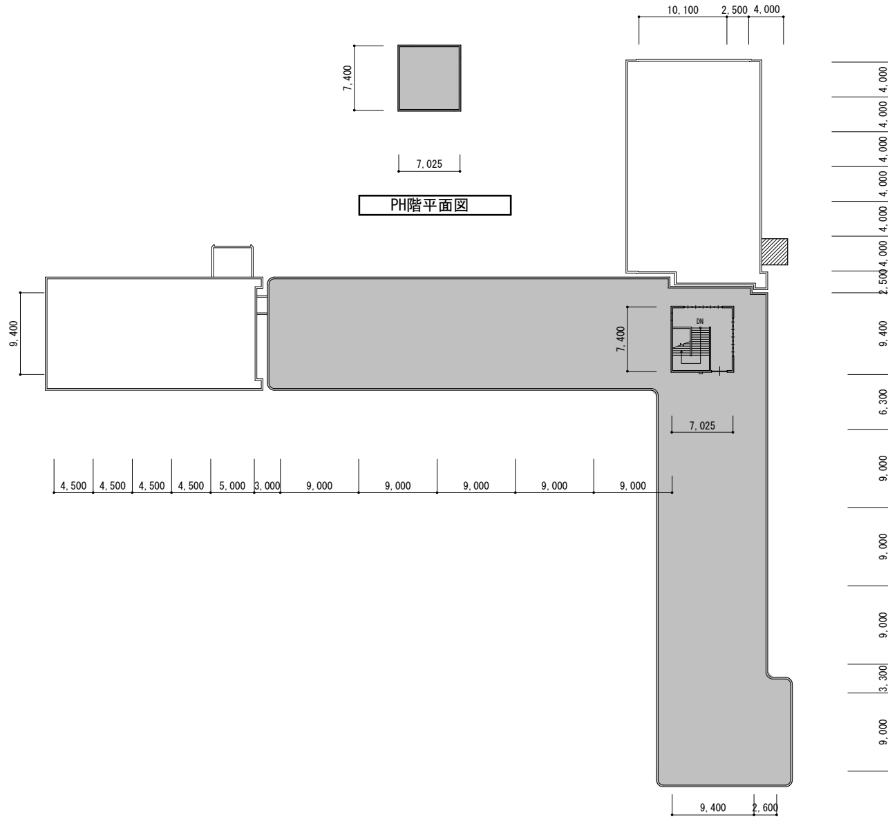
屋上階平面図
