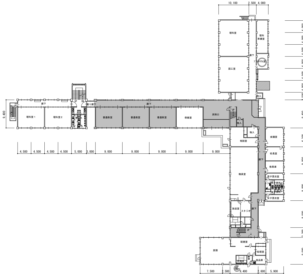
1階平面図
