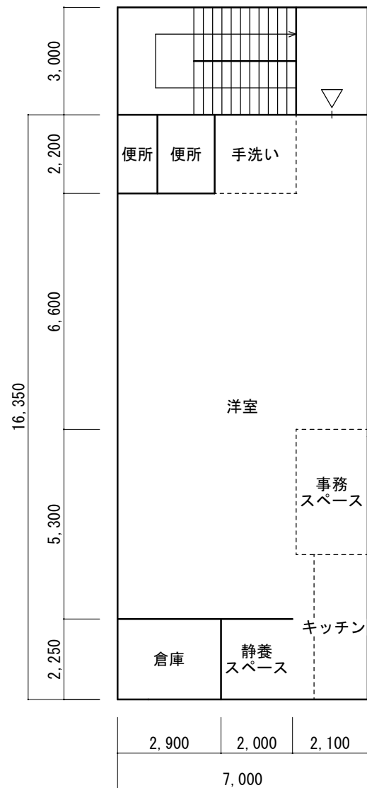
2 階平面図 (参考)
