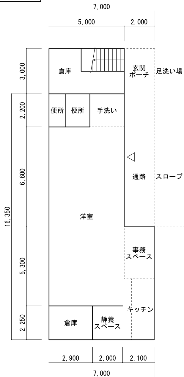
1 階平面図 (参考)
