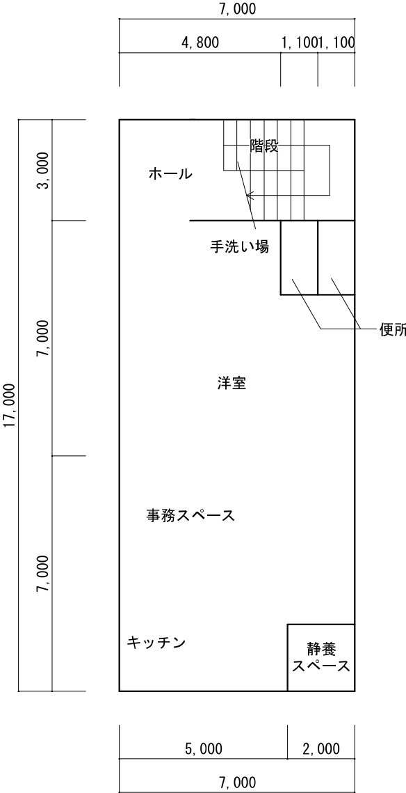
2 階平面図 (参考)
