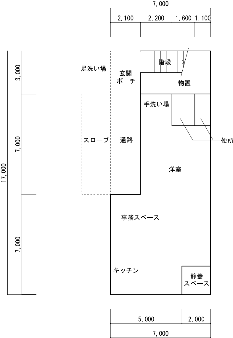
1 階平面図 (参考)
