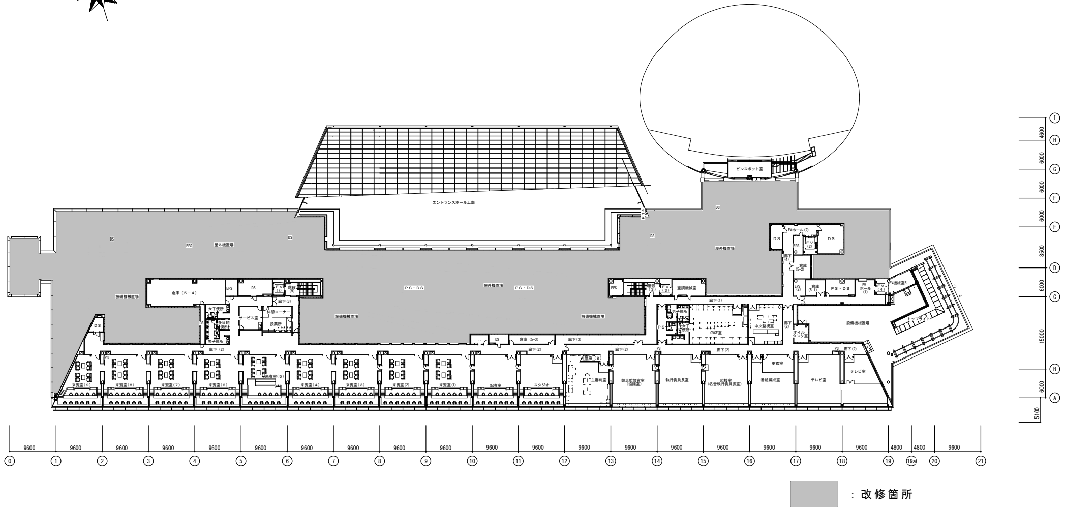
5 階平面図
