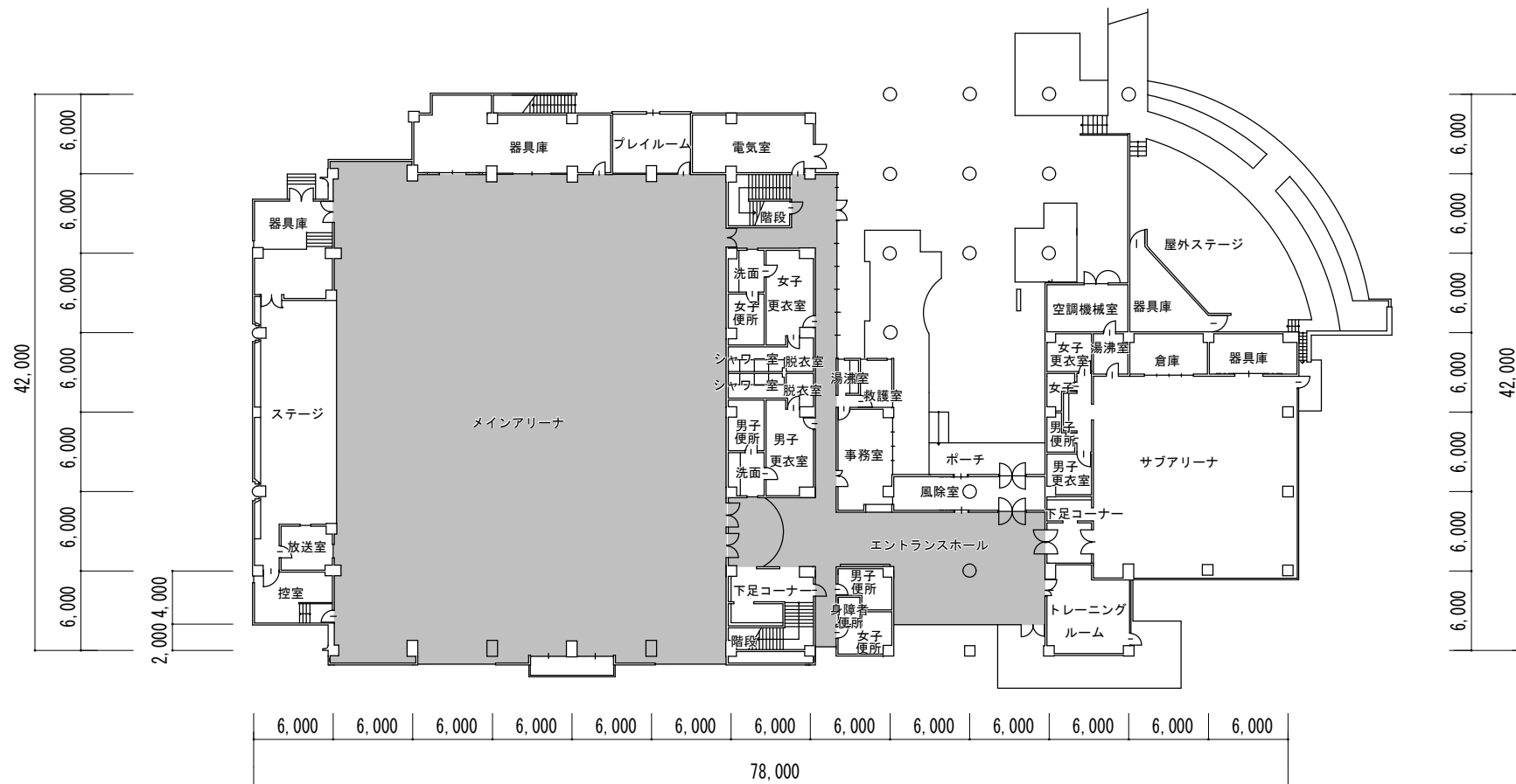
1階平面図
