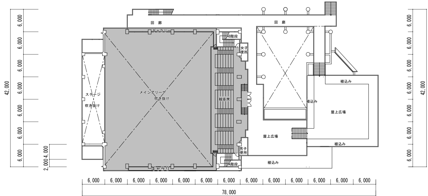
2階平面図
