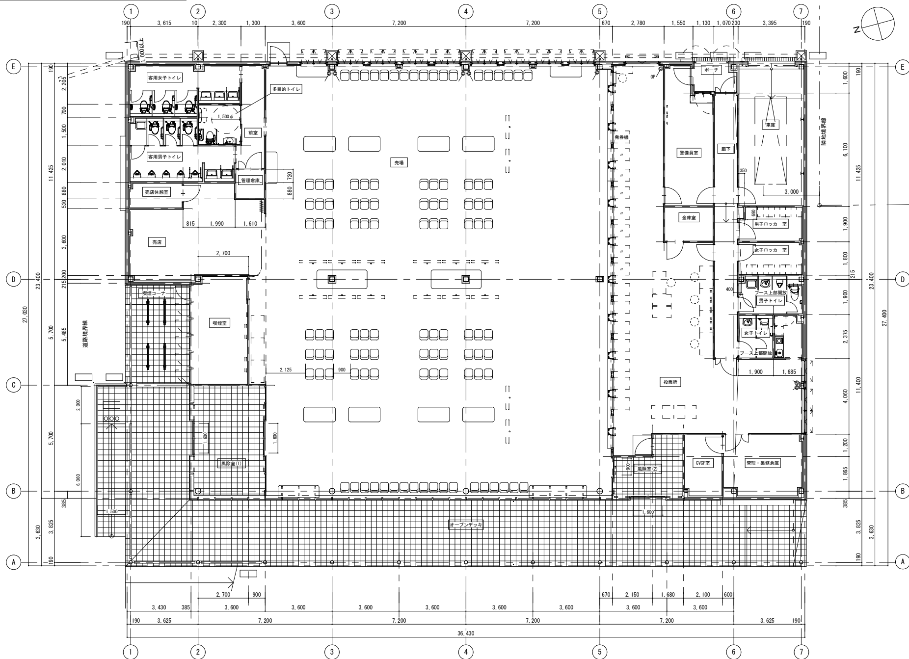
1 階平面図
