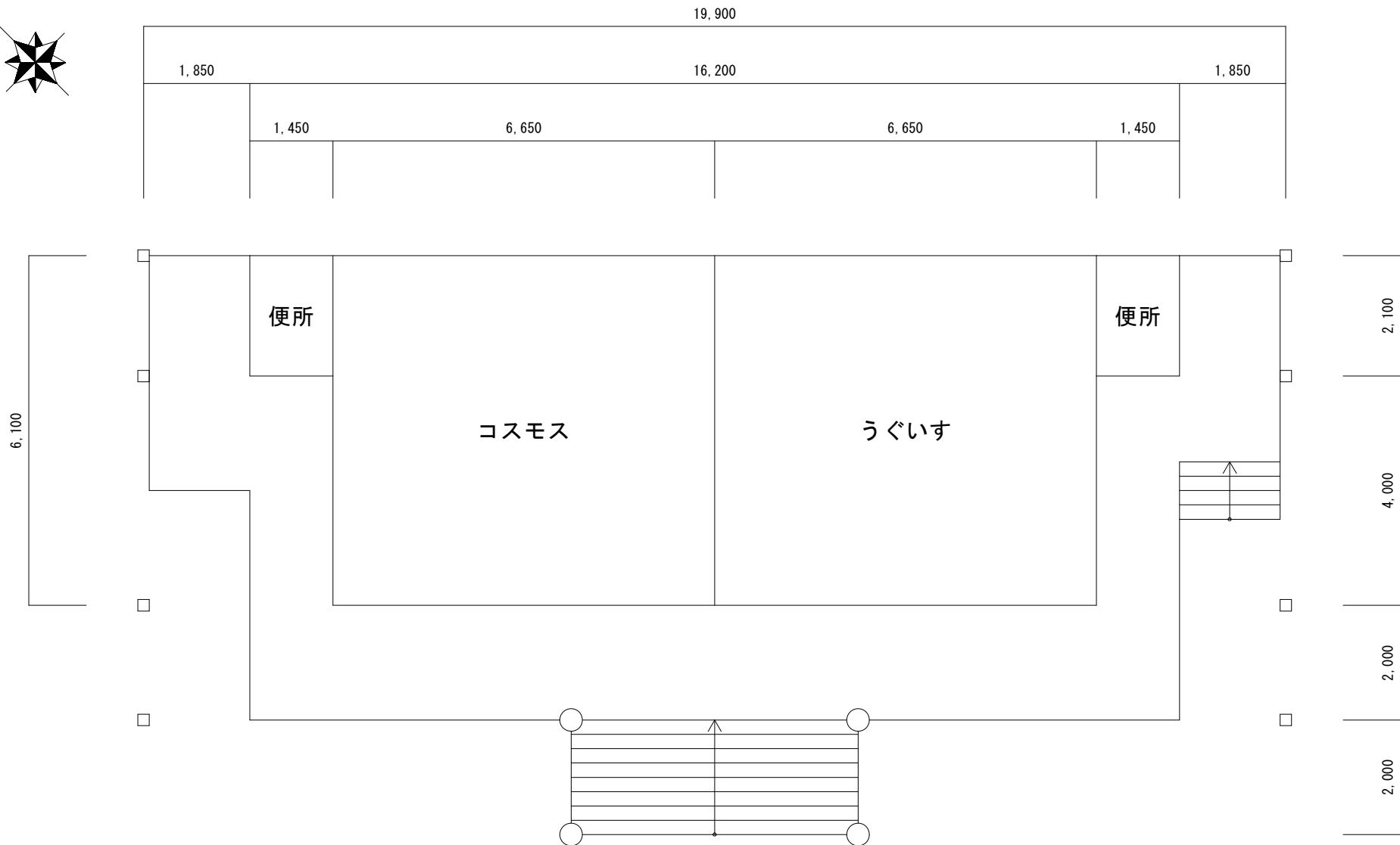
平面図
