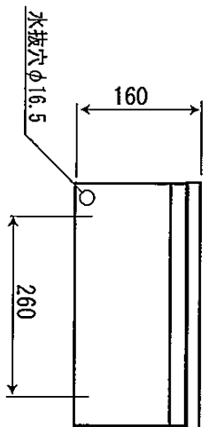
底面図
