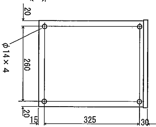
背面図
