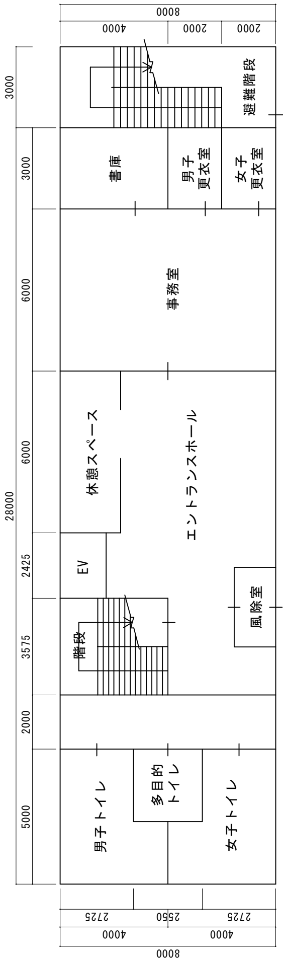
1 階平面図（参考）
