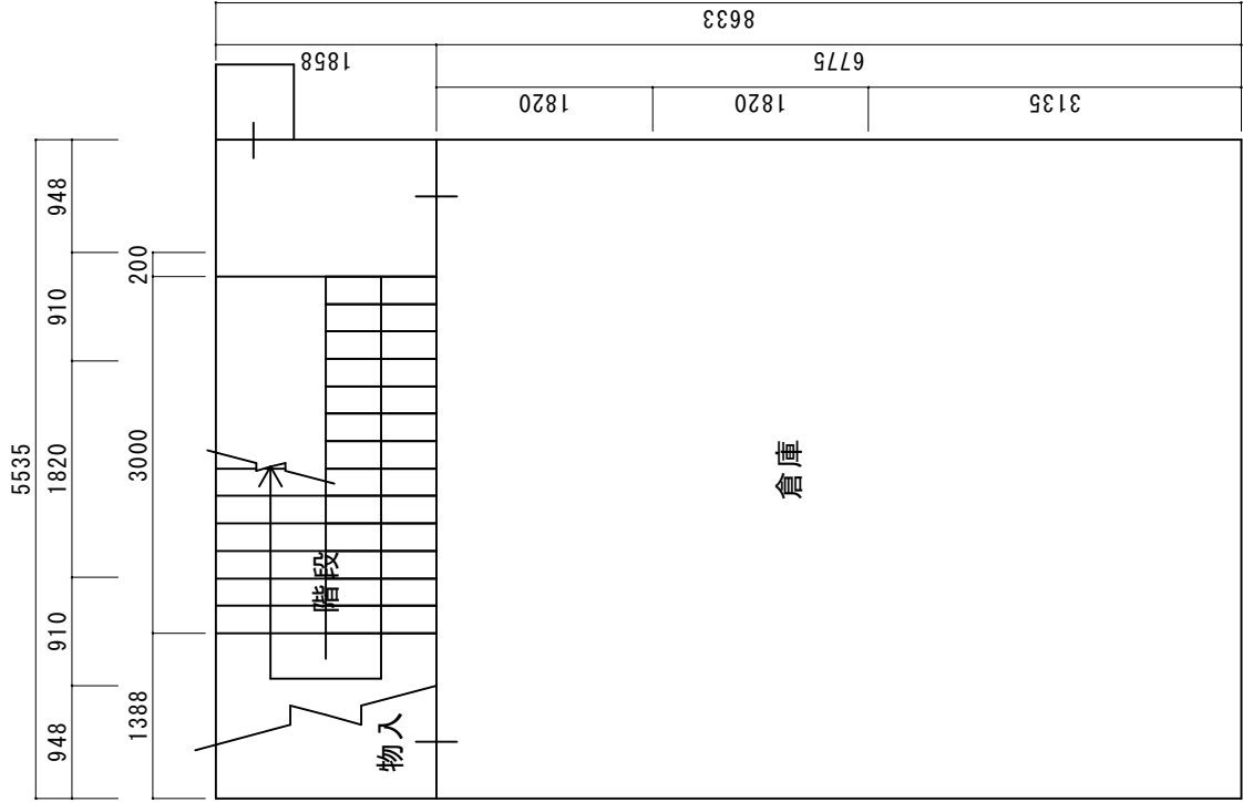
1 階平面図 (参考)
