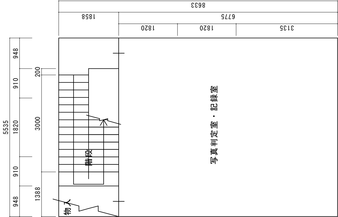
2 階平面図 (参考)
