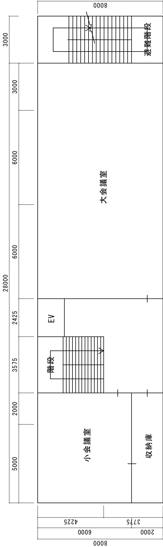
1 階平面図（参考）
