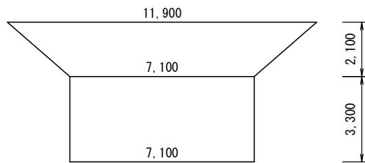
すりつけ部① No. 12+34. 6付近(右)
