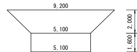
すりつけ部③ No. 13+31. 6付近(右)
