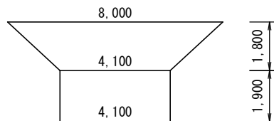
すりつけ部④ No. 14+27. 6付近(右)
