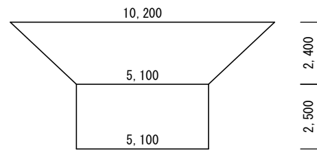
すりつけ部② No. 12+34. 6付近(左)
