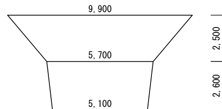
すりつけ部⑤ No. 15+32. 6付近(左)
