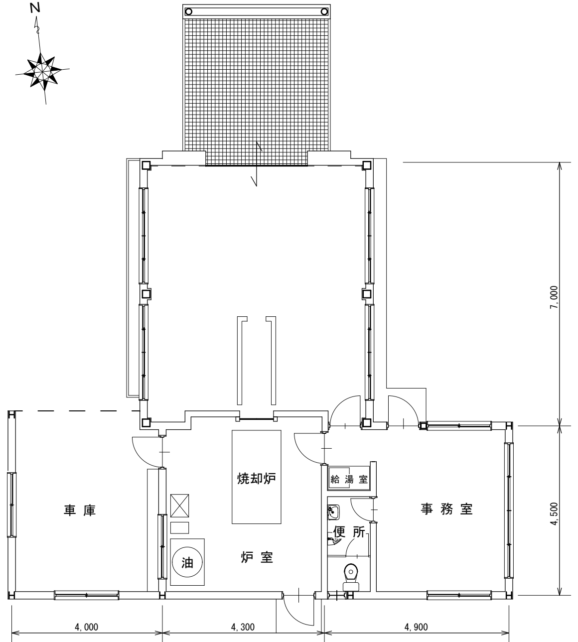
平面図 S=1/100
