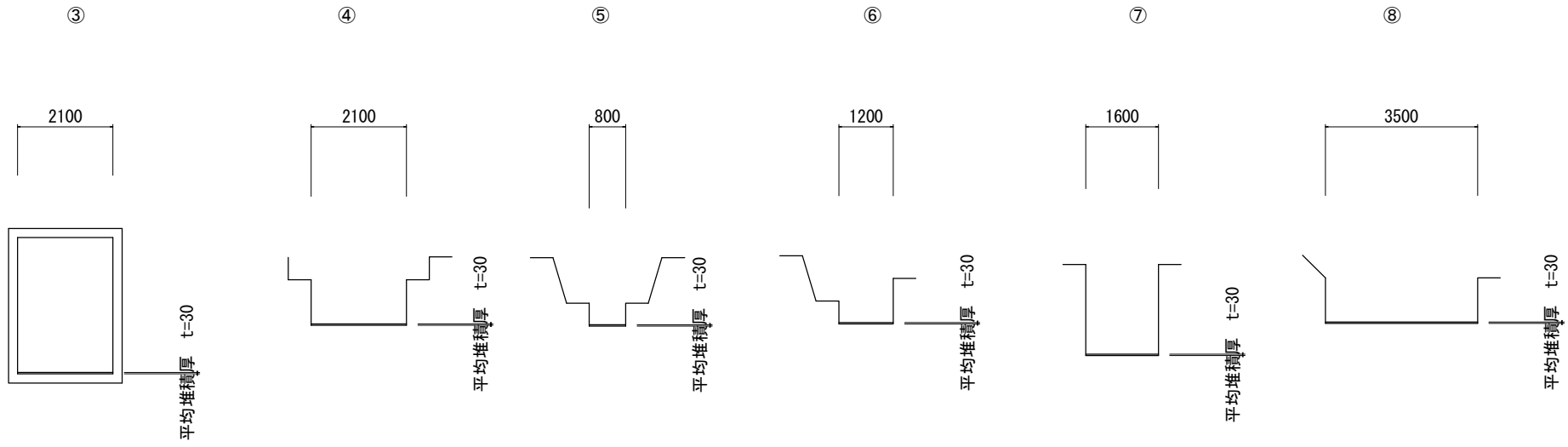
断面图 (2)
