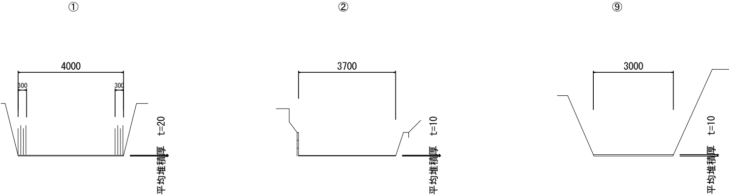
断面图 (1)
