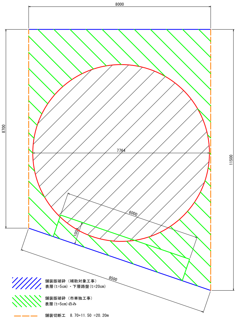
舗装撤去復旧工 平面図
