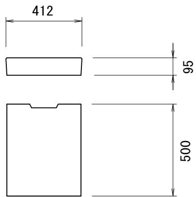
側溝蓋 (1)
