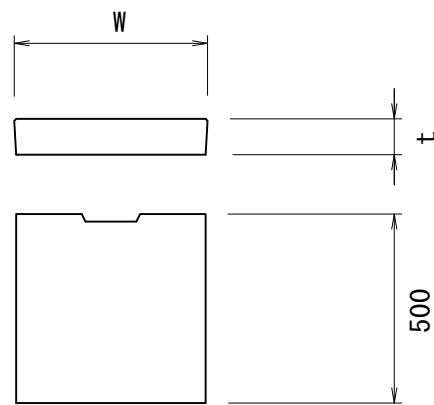
側溝蓋 (2) (3)
