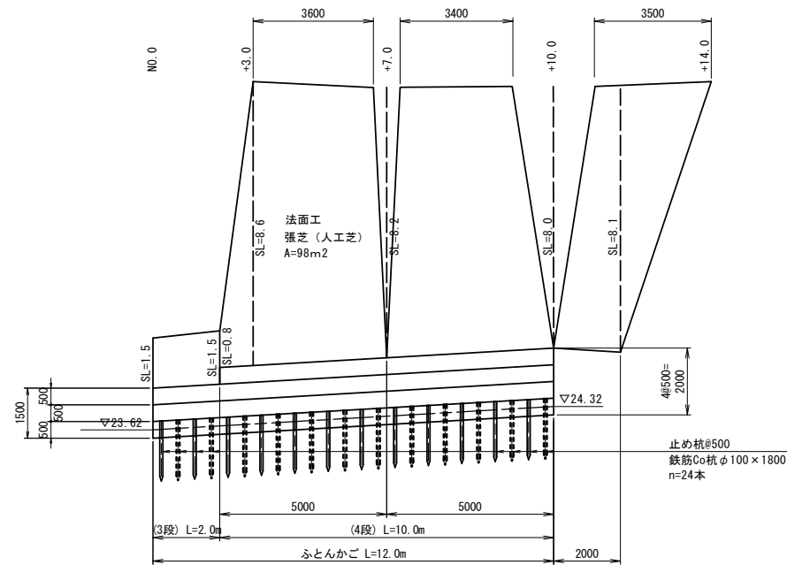
展開図 S=1:100
