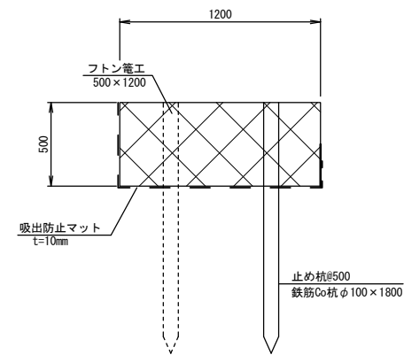
工法図 S=1:20
