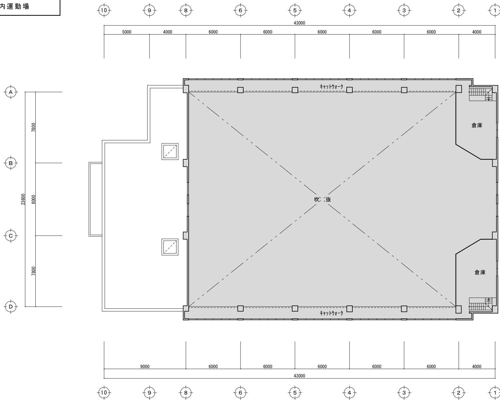
2階平面図
