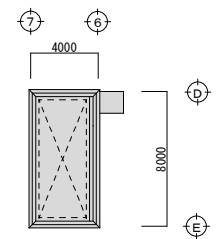
PHR階平面図
