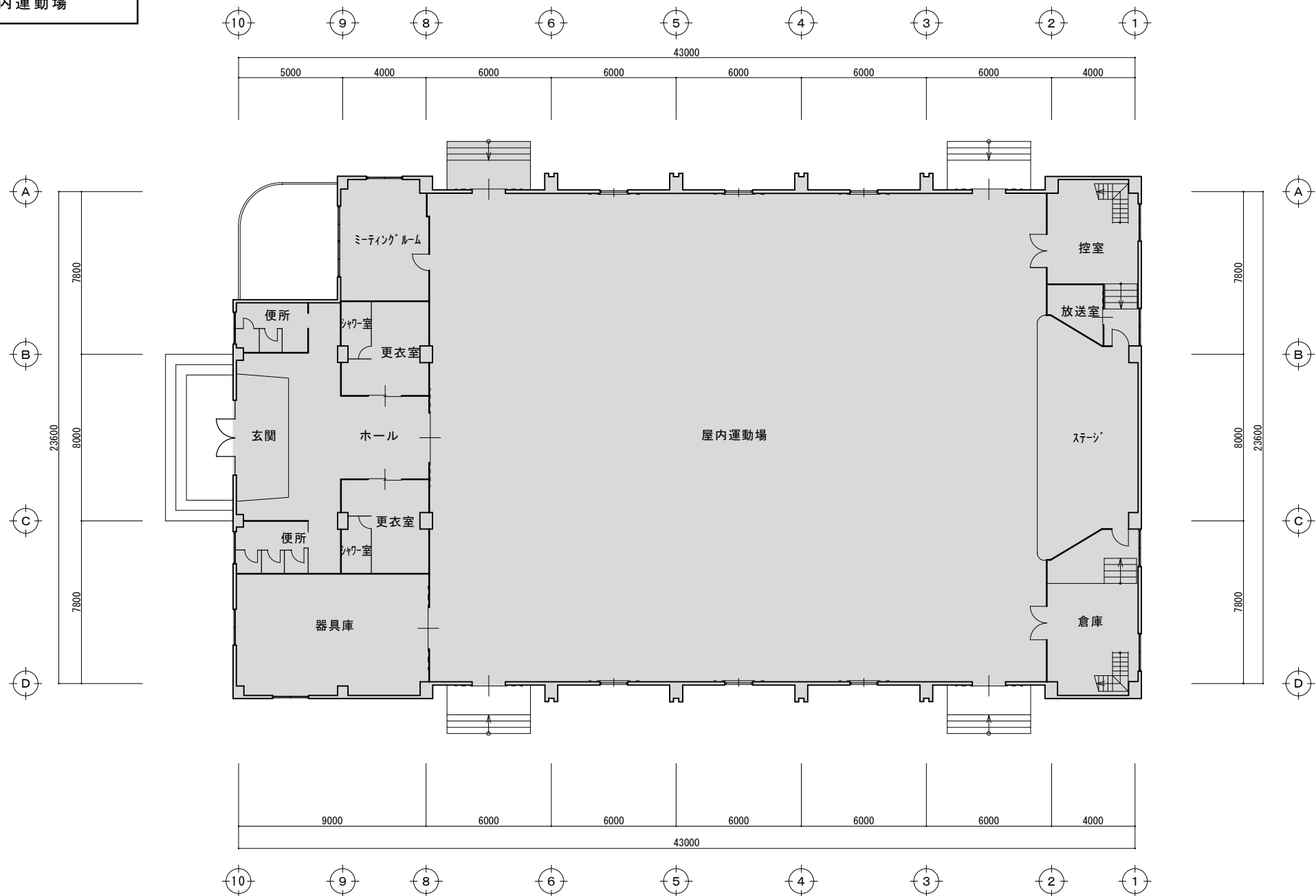
1階平面図
