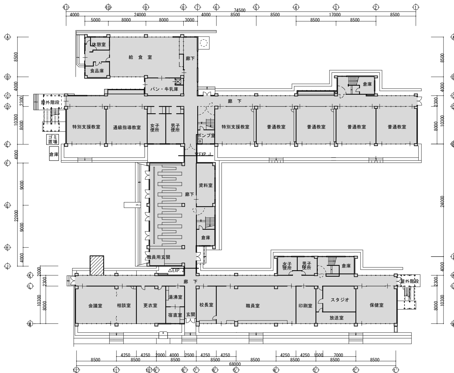
1階平面図
