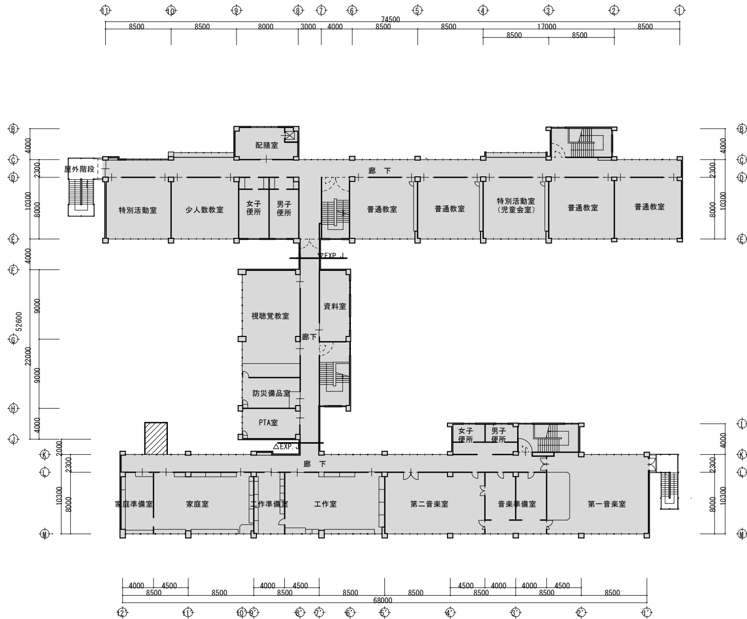
3階平面図
