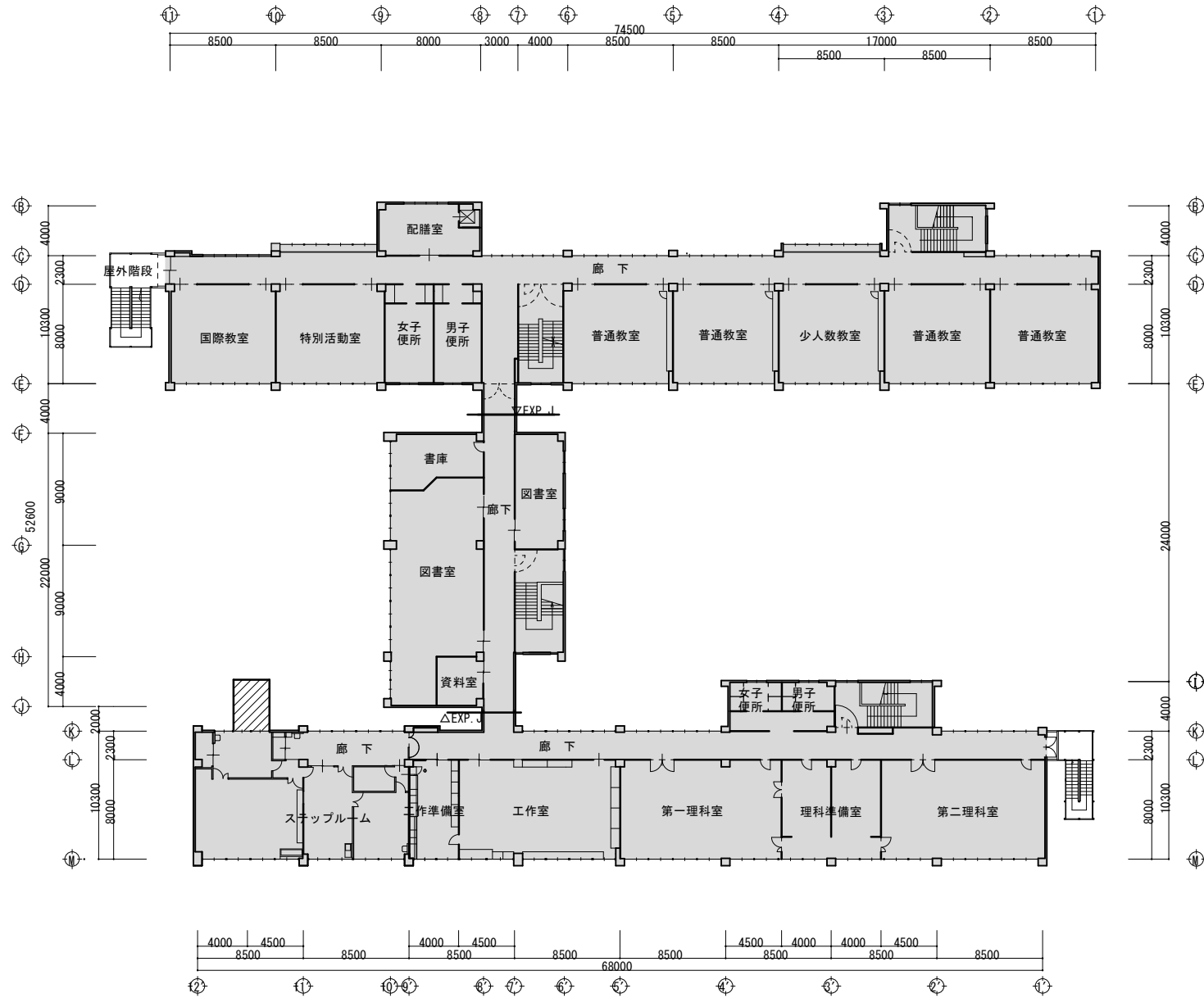
2階平面図
