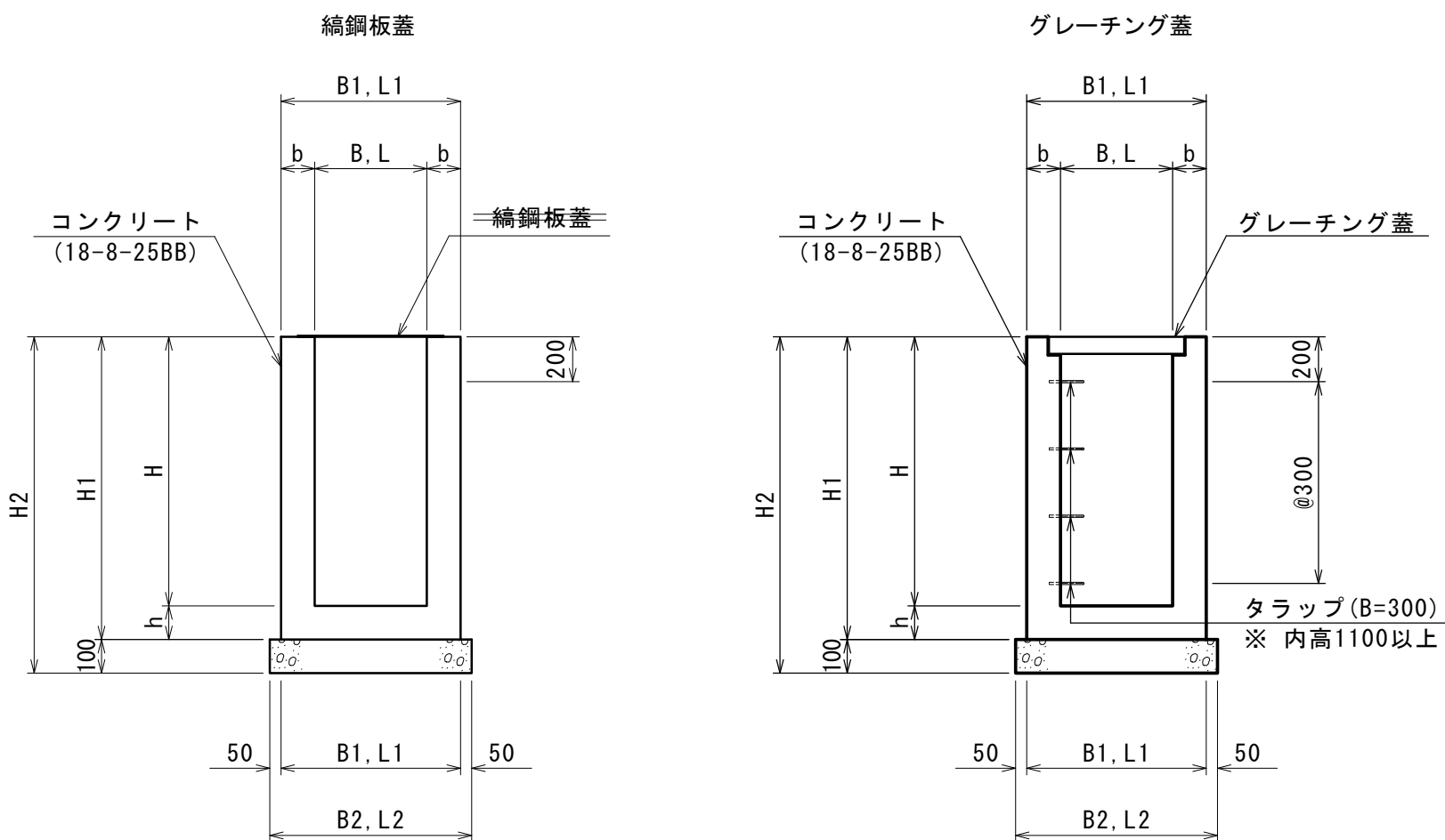
断面図
