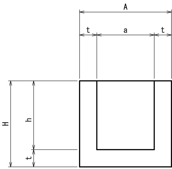
集水樹寸法表
