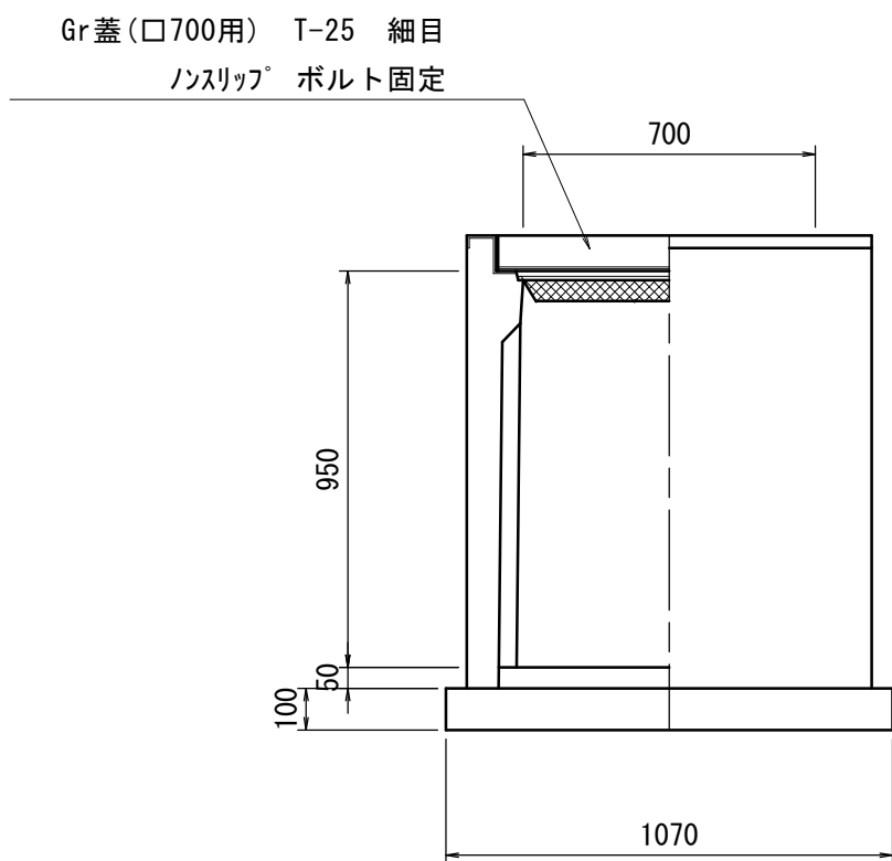
断面図
