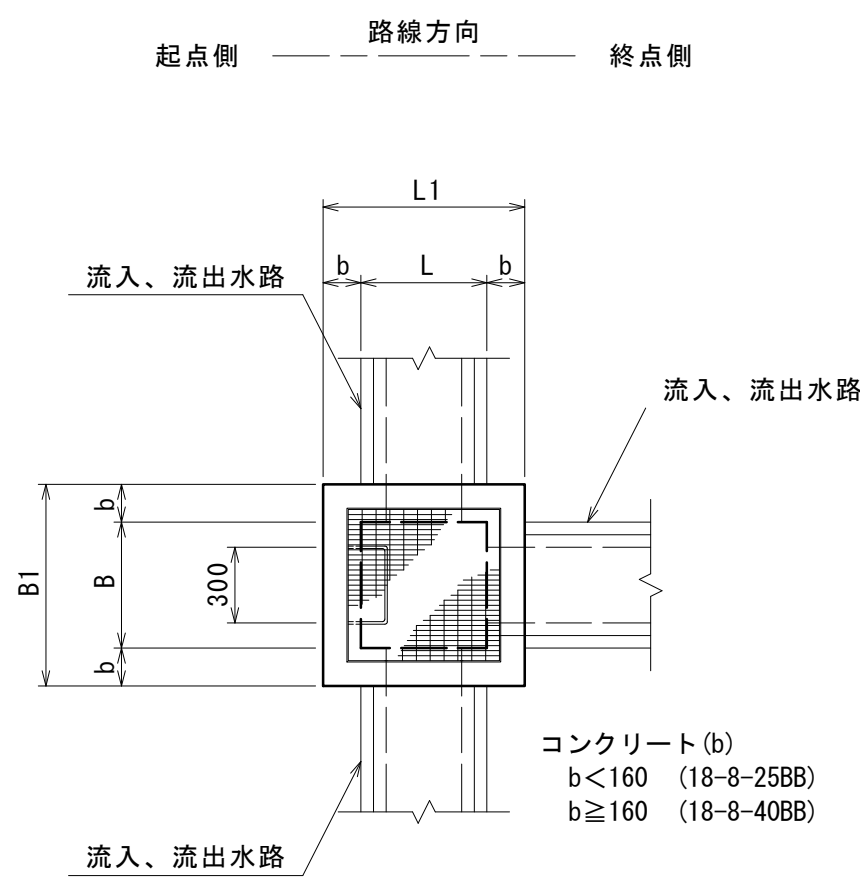
平面図
