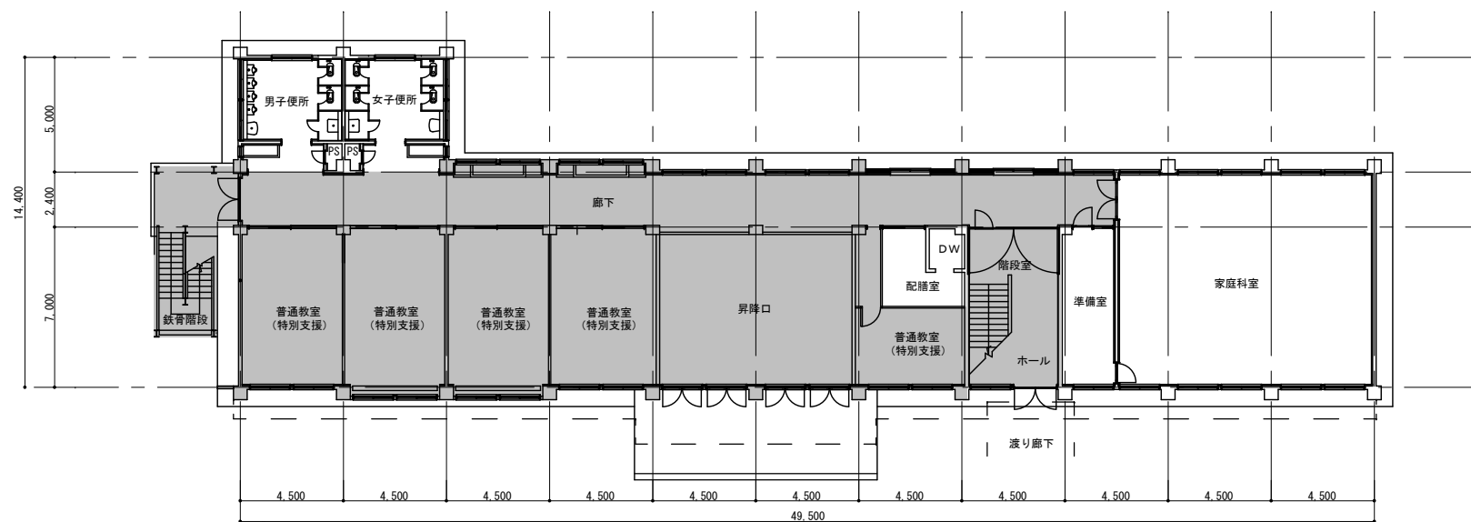
1 階 平 面 図
