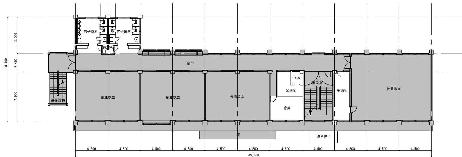
2 階 平 面 図
