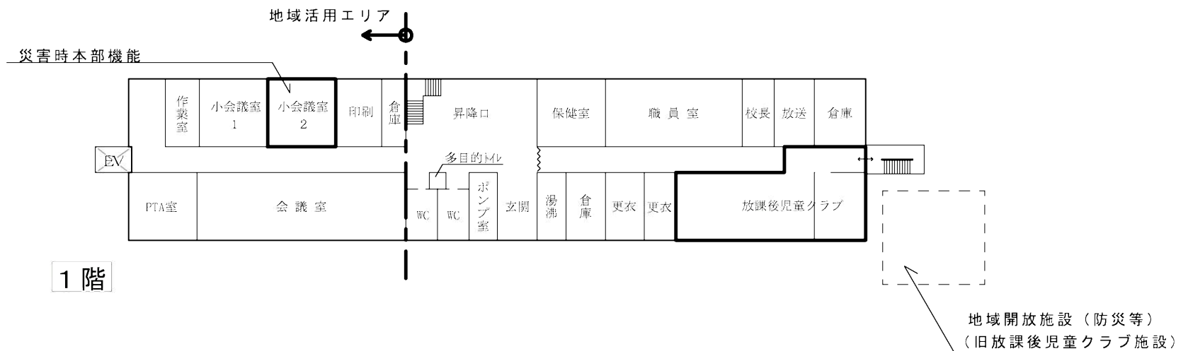
特別教室管理棟 1、2 階平面図
