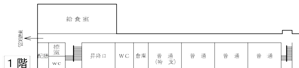
普通教室棟 1 ～ 3 階平面図
