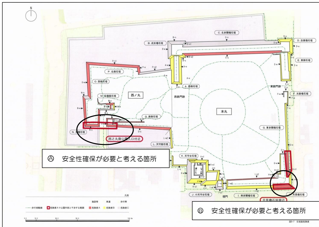
津城跡石垣の傷み状況把握図
