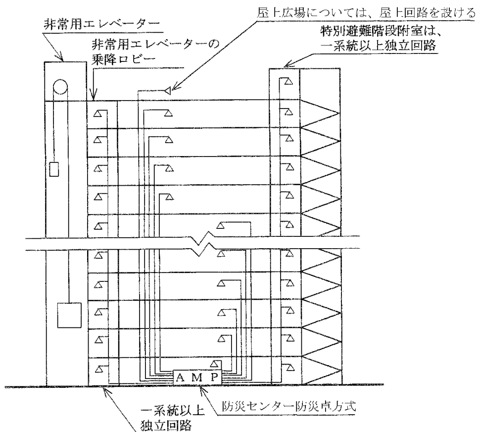
例図6 放送設備
