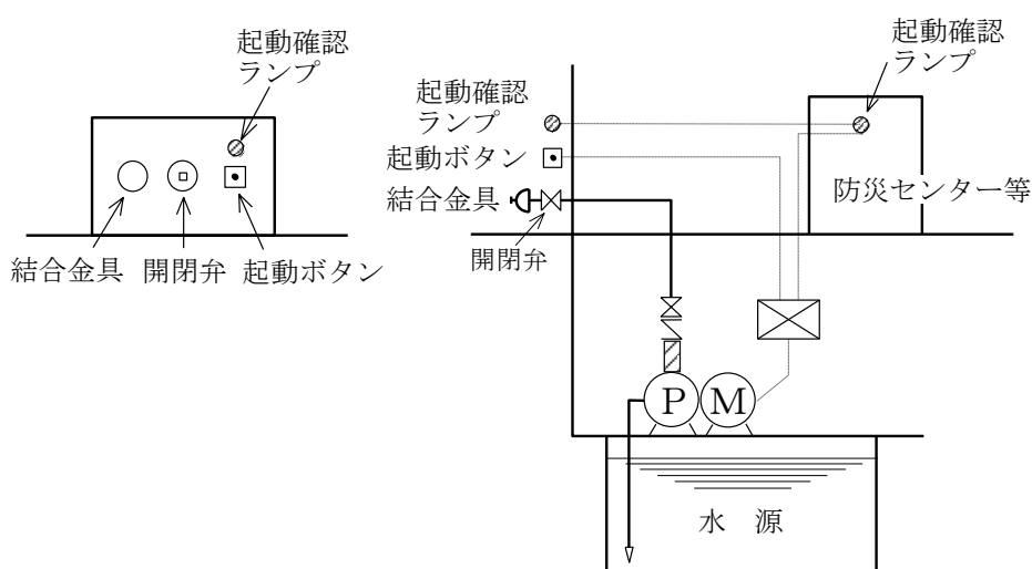
第18-2図 a 結合金具直近からの遠隔起動の場合
