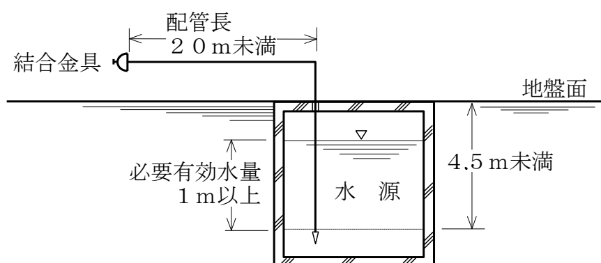
第18-1図 b 結合金具より下の水源を有する消防用水
