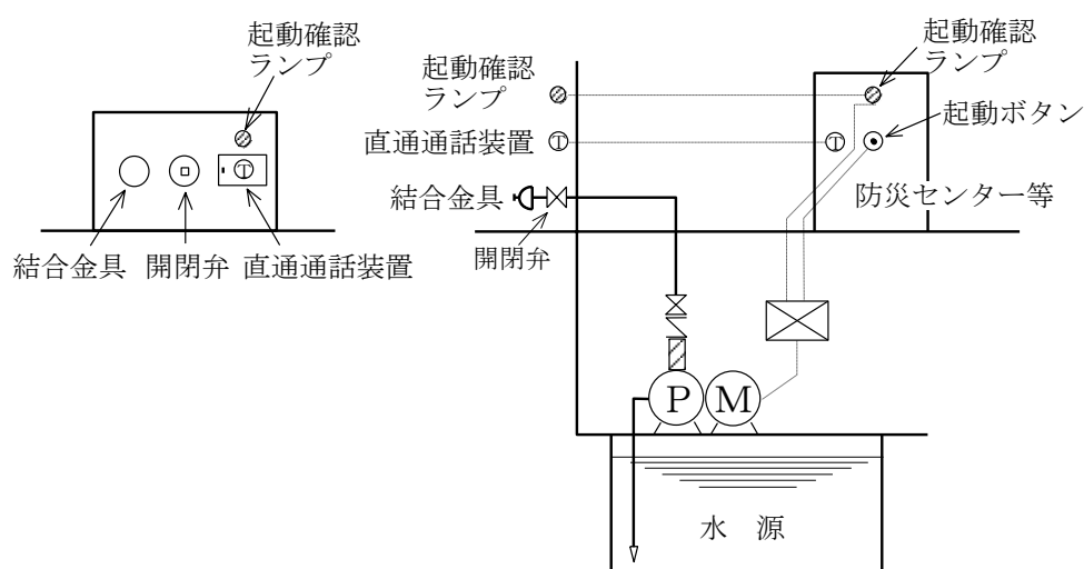
第18-2図 b 防災センター等からの遠隔起動の場合
