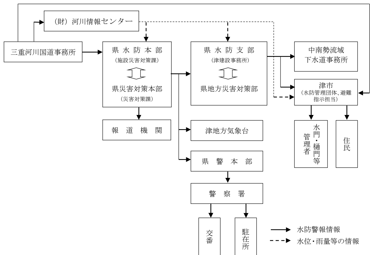
d 水位情報の通信連絡系統図（図2）
