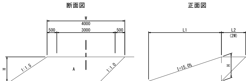
仮設構造図
