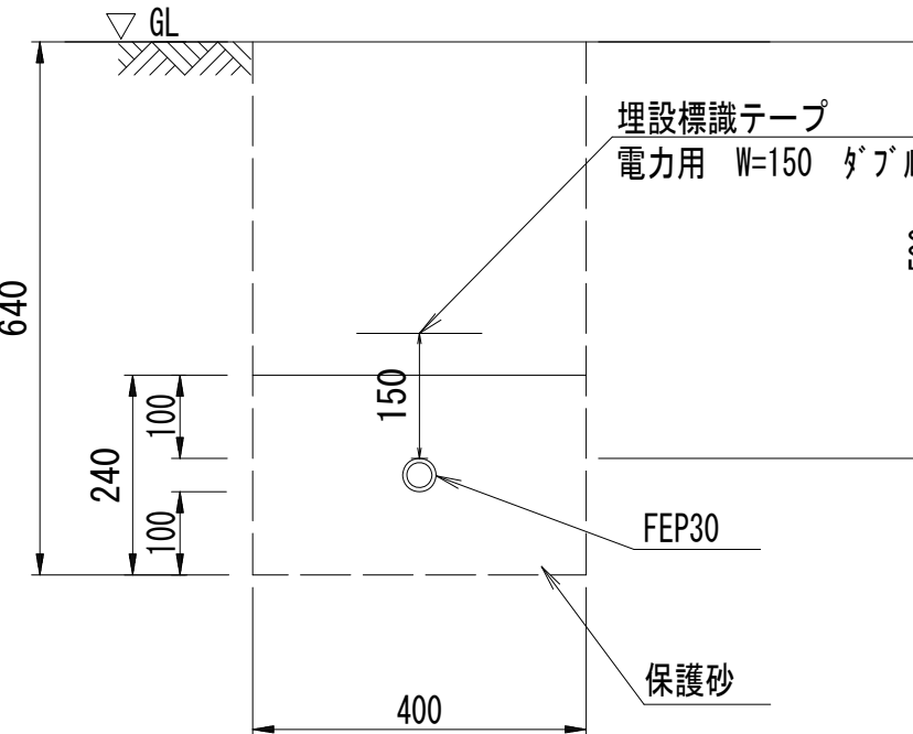
電線管 S=1:
