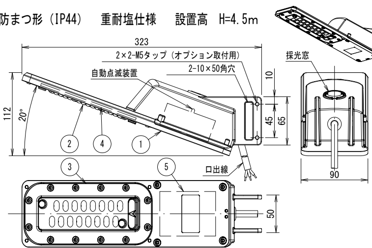
照明器具姿図 E70073SAN9 (同等品以上) S=1:5
